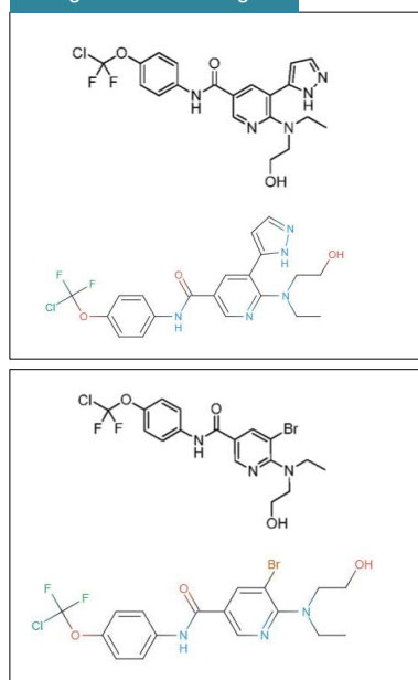
Deep Parsing
