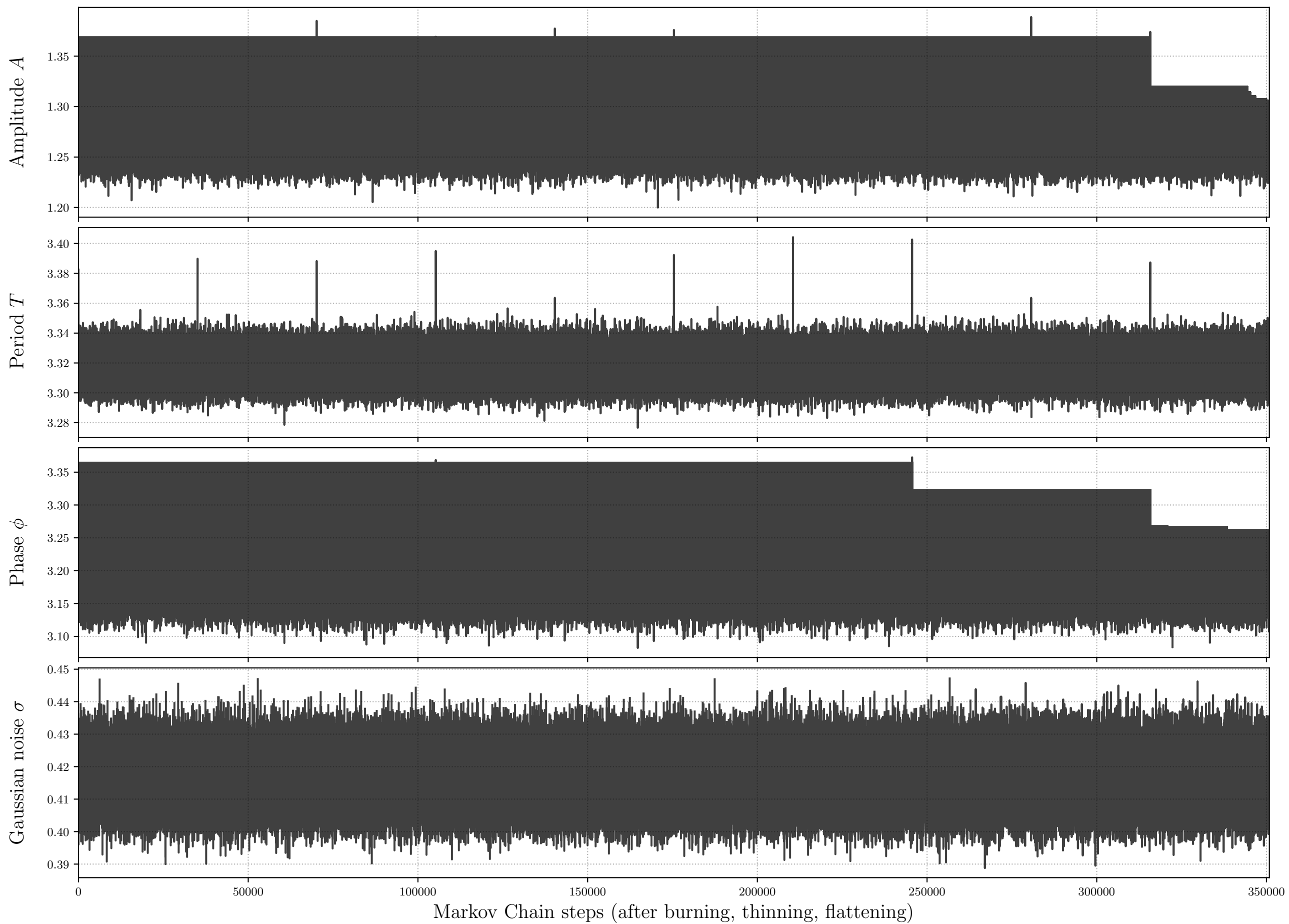
Monte Carlo Markov Chain, Parameters A, T, \phi, \sigma :
