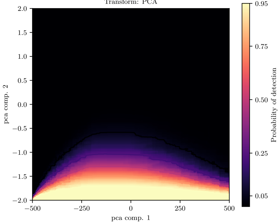
Transform: PCA
