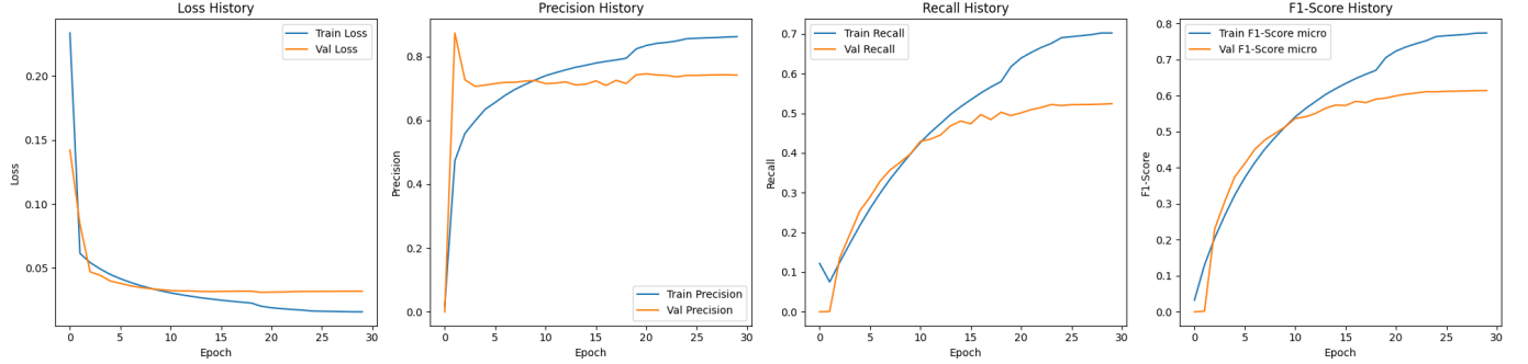
Figure 13: Curve di validazione e training di Loss, Precision, Recall e F1-Score(da sinistra a destra).
