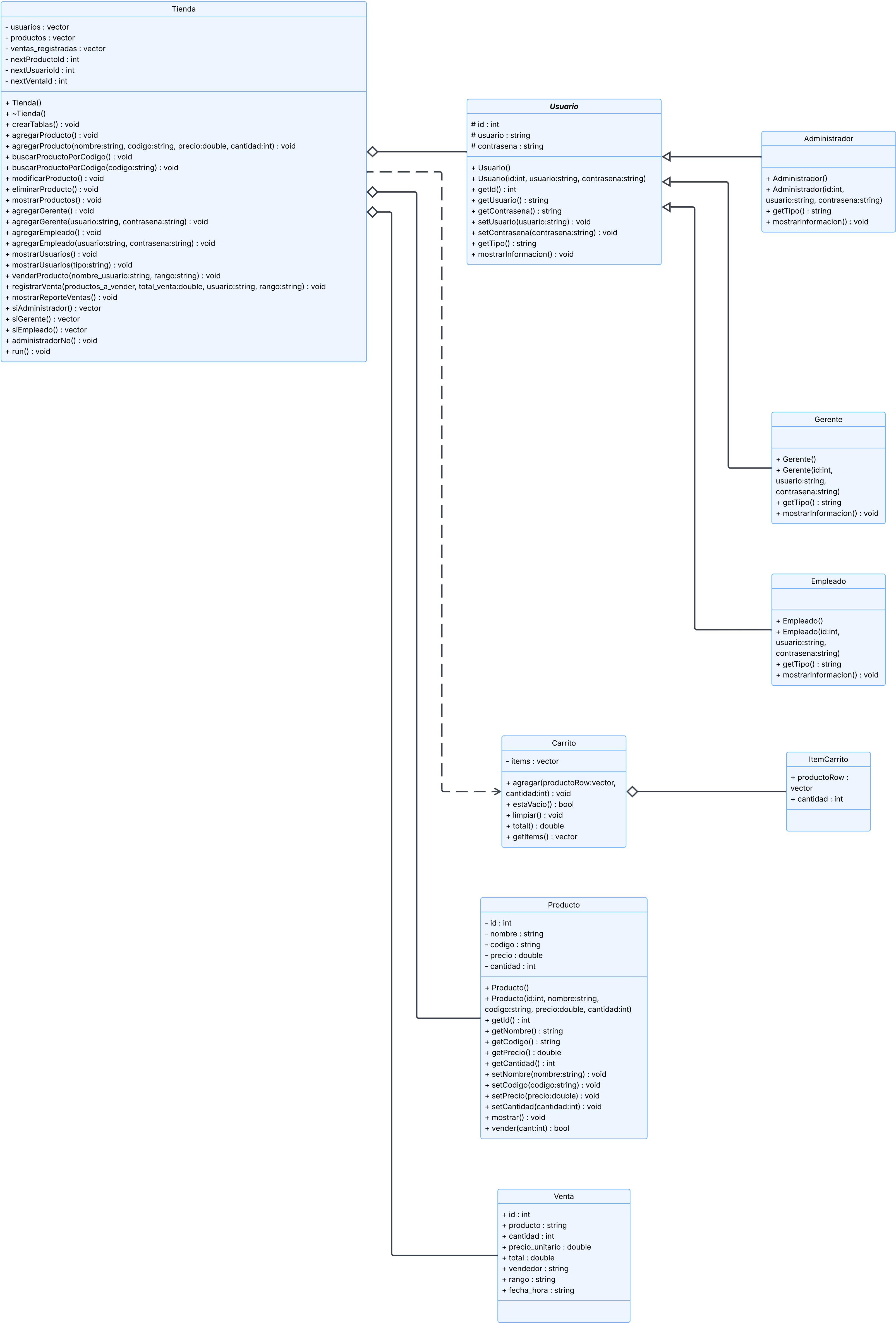
Diagrama de Clases: Tienda
