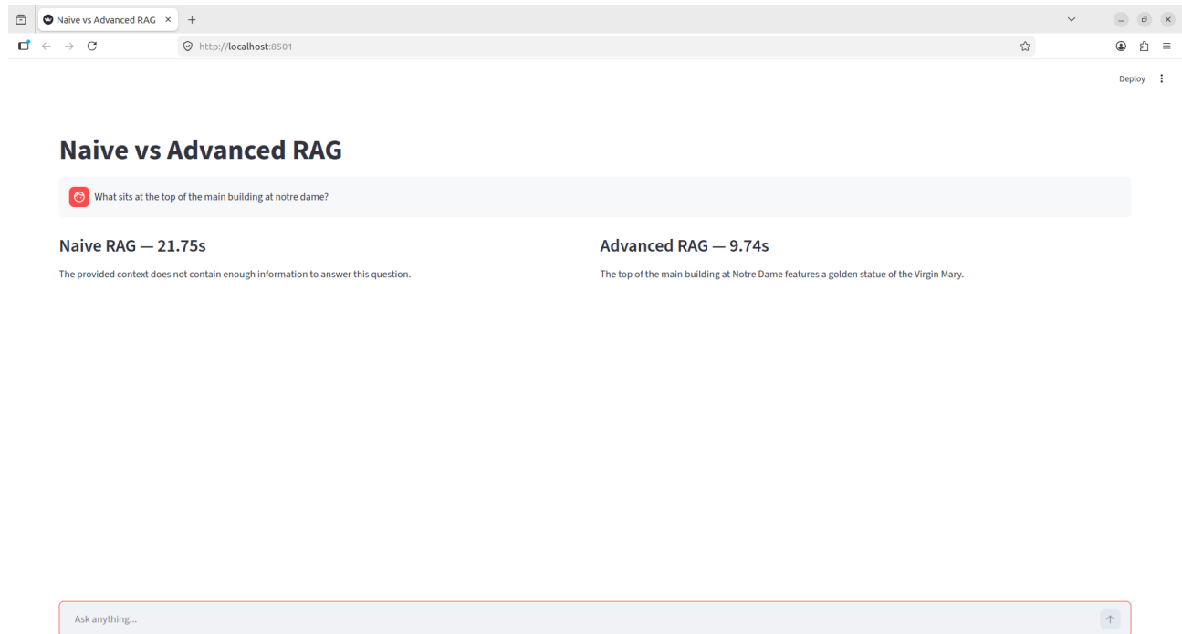
Figura 3.11: Interfața comparativă a demonstratorului. Cele două coloane corespund pipeline-urilor Naive și Advanced, care răspund simultan la aceeași întrebare, cu timpii de generare afișați deasupra fiecărui răspuns. În acest exemplu, Naive RAG nu găsește răspunsul, în timp ce Advanced RAG recuperează fragmentul corect.
