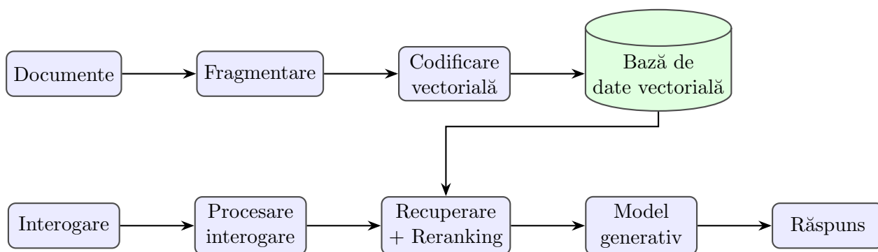
Figura 1.3: Arhitectura generală a unui sistem RAG: indexare offline (sus) și inferență online (jos) [6, 23].
