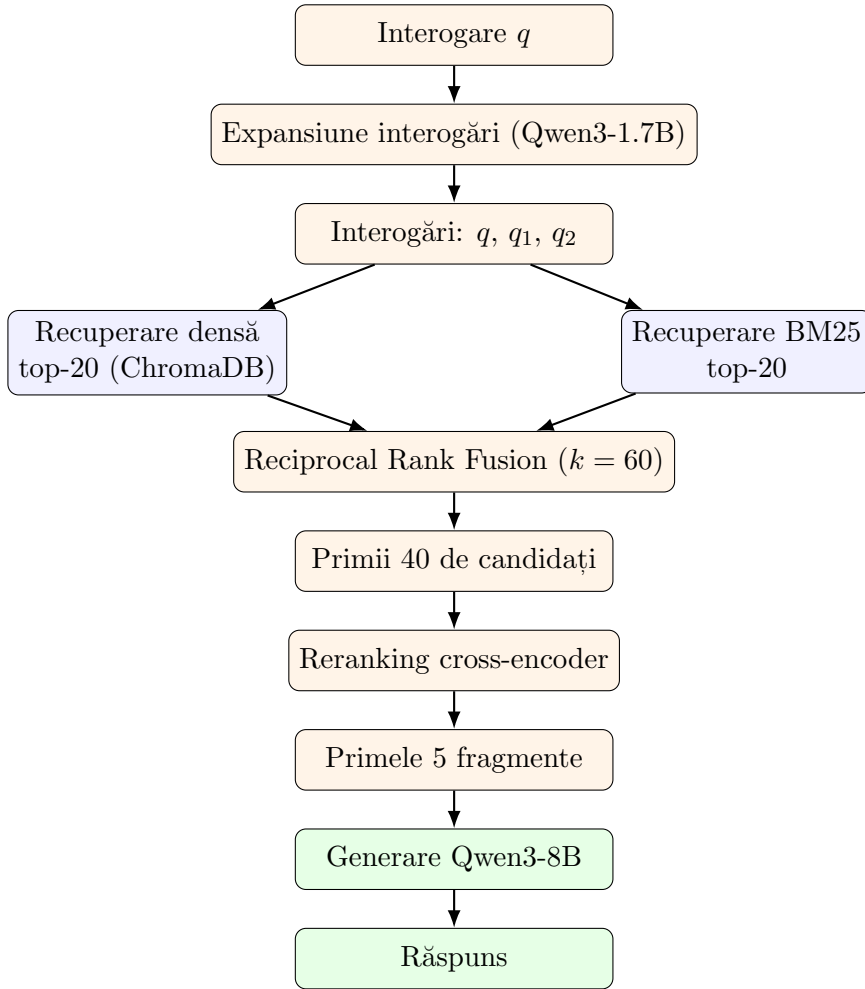
Figura 2.3: Fluxul de procesare Advanced RAG. Interogarea este reformulată, fiecare variantă este căutată dens și prin BM25, rezultatele sunt fuzionate prin Reciprocal Rank Fusion, rescorate cu un cross-encoder, iar primele cinci fragmente sunt trimise modelului generativ.
