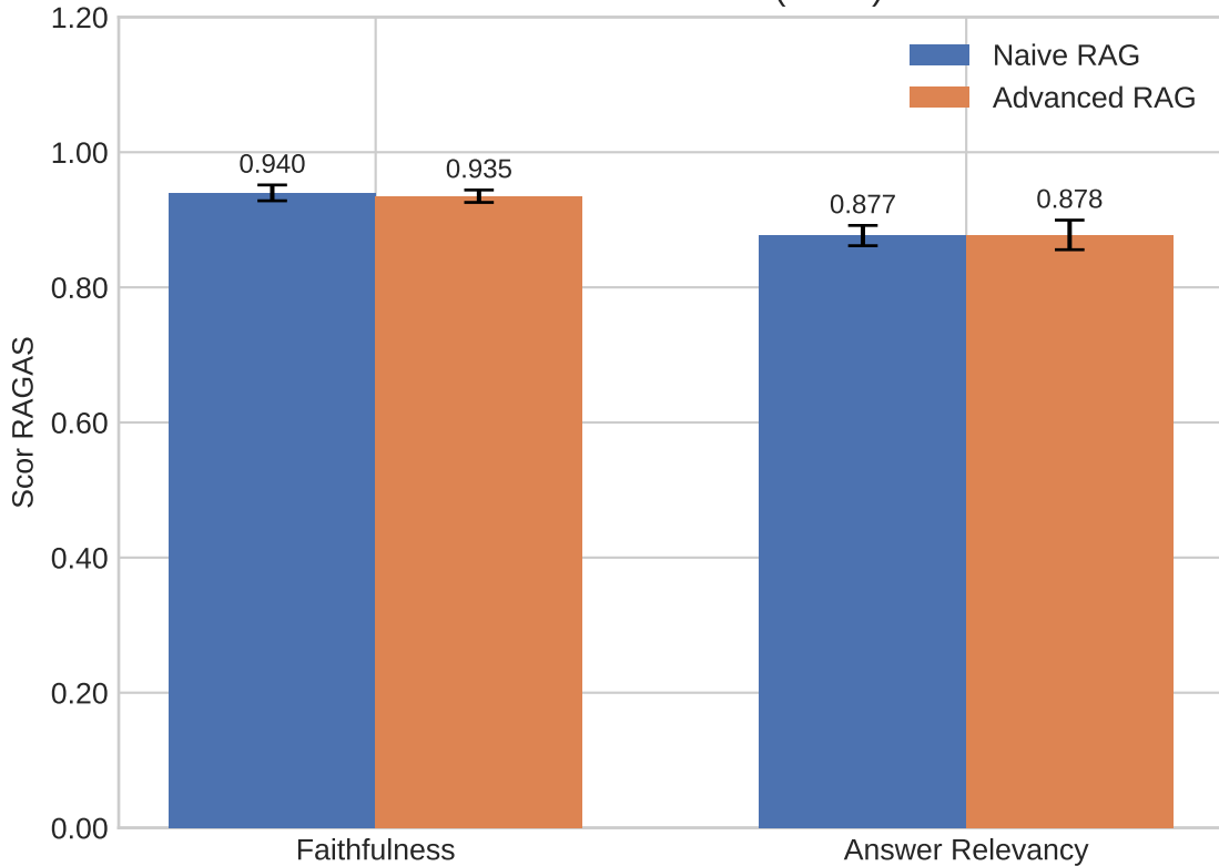
Metrici RAGAS — subset comun (N=70) — DOCRED
