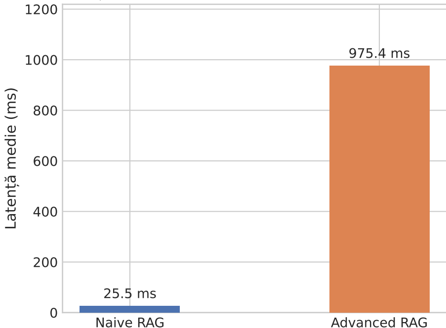
Latența Medie de Procesare a Interogării — SQUAD
