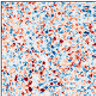
conv 1×2
