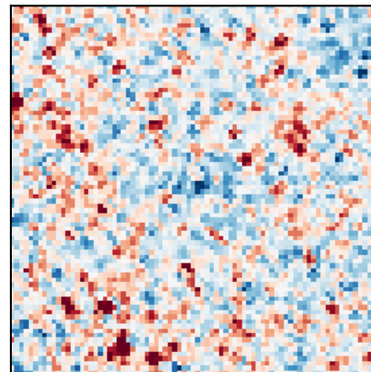
conv 2×3
