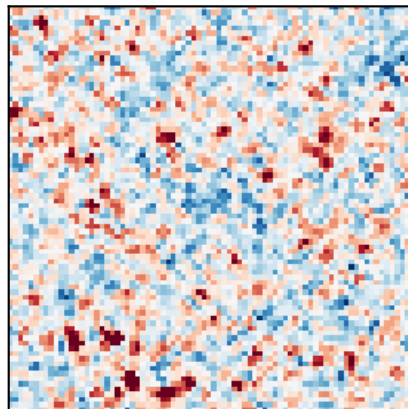
conv 1×4
