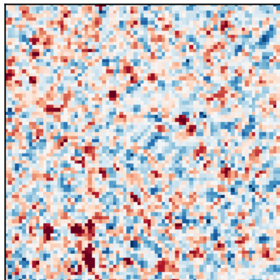
conv 1×3
