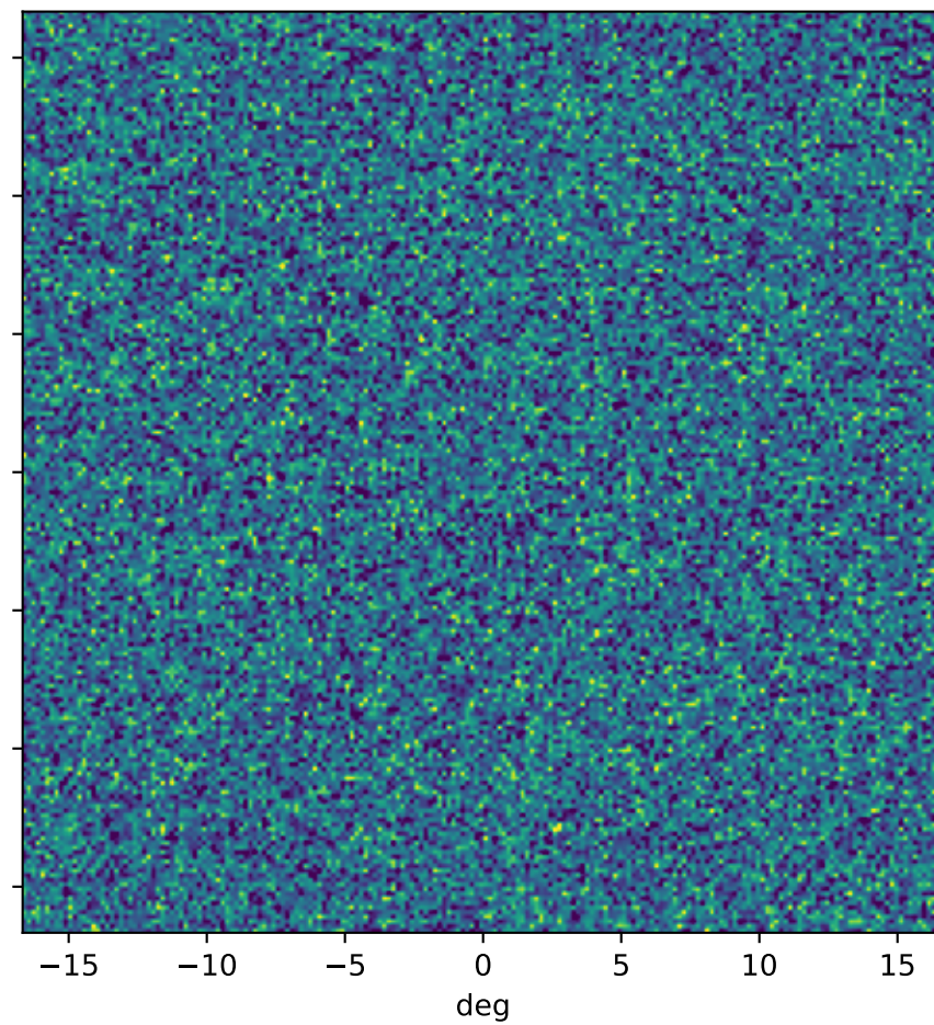
BNT bin 2
