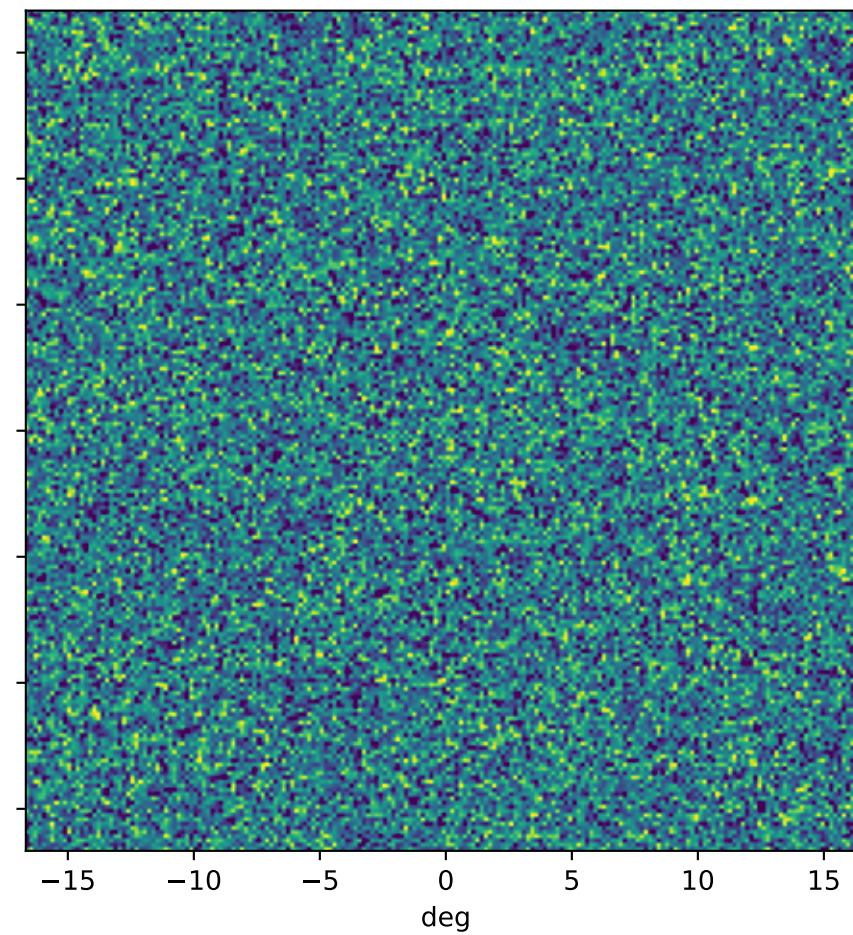
BNT bin 4
