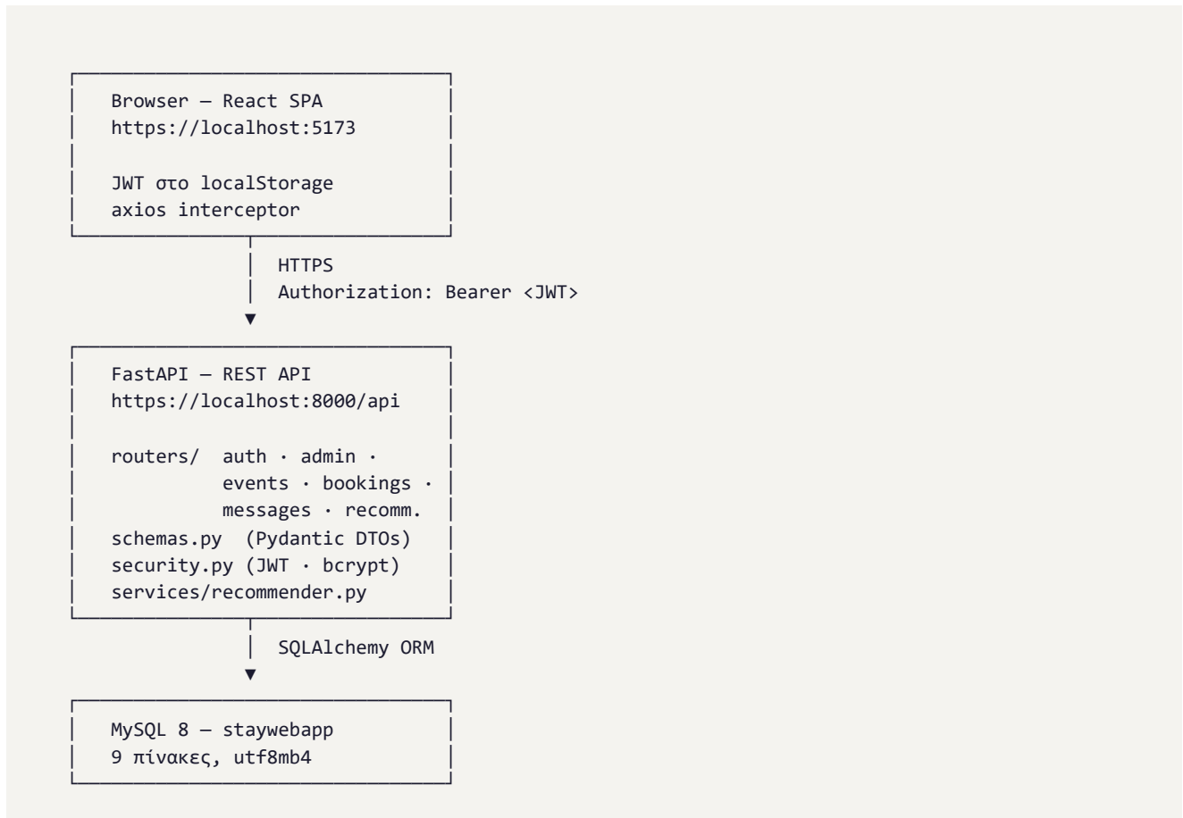
Σχήμα 2.1 — Τα τρία επίπεδα της εφαρμογής.
