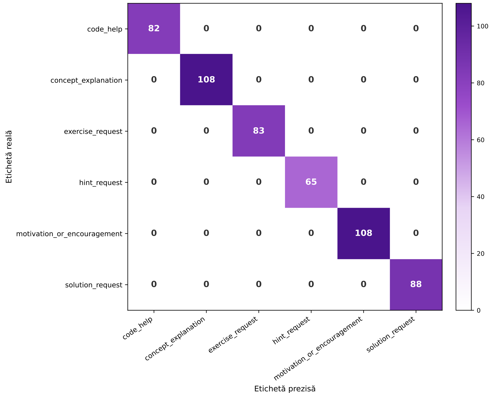
Ensemble BERT v2 + XLM-R v2 — Label Avg. Probabilities | Acc=100.00% F1=100.00%
