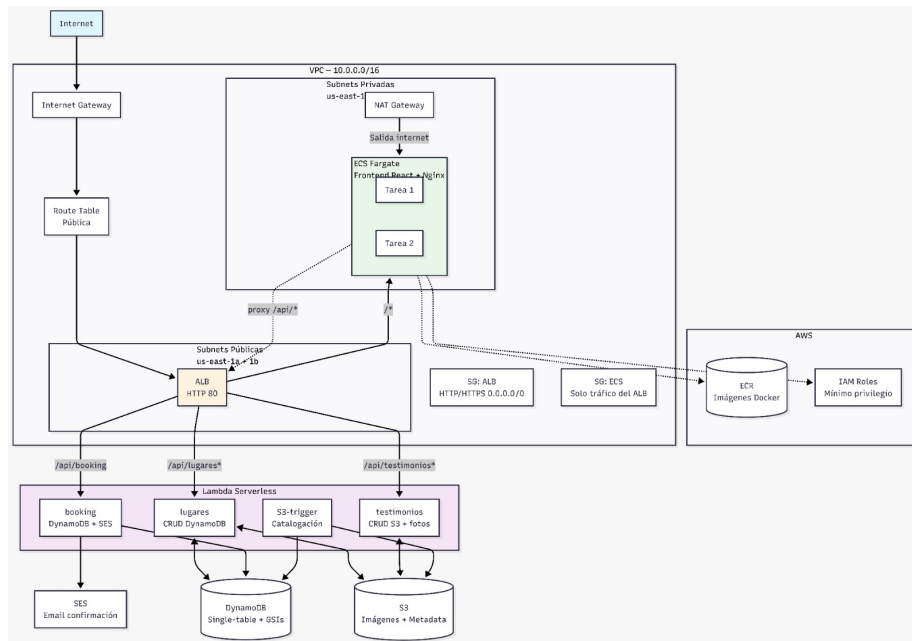
Figura 1: Diagrama de la infraestructura
