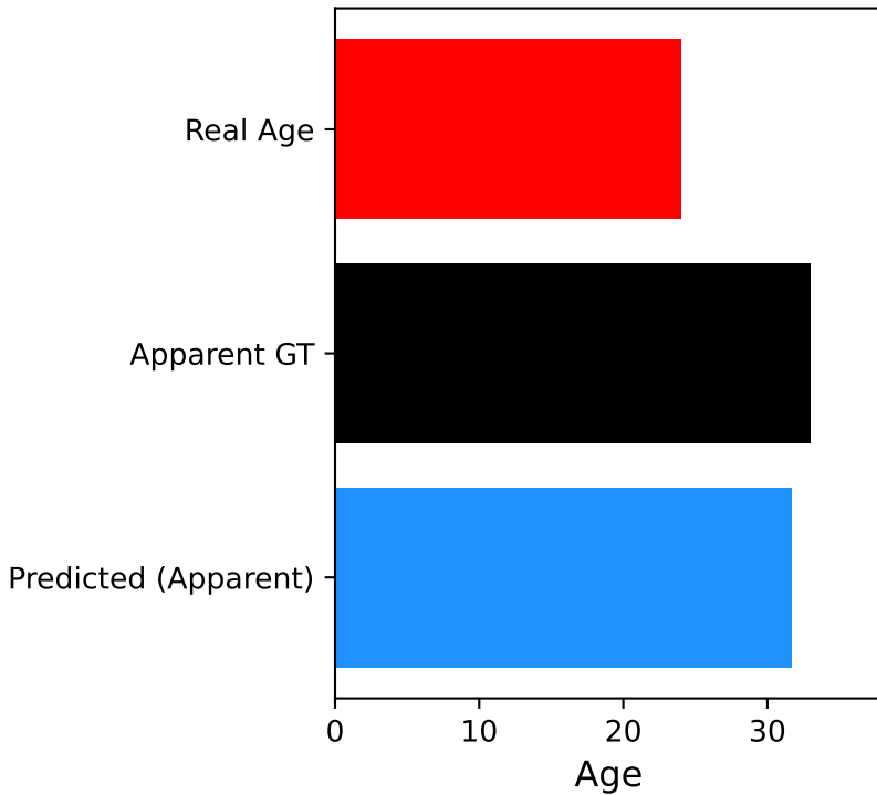
ID: 007409.jpg
