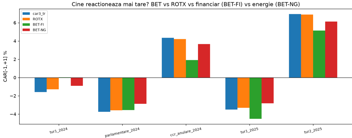
Figura 2: CAR[-1, +1] pe indici la cele cinci șocuri majore.
