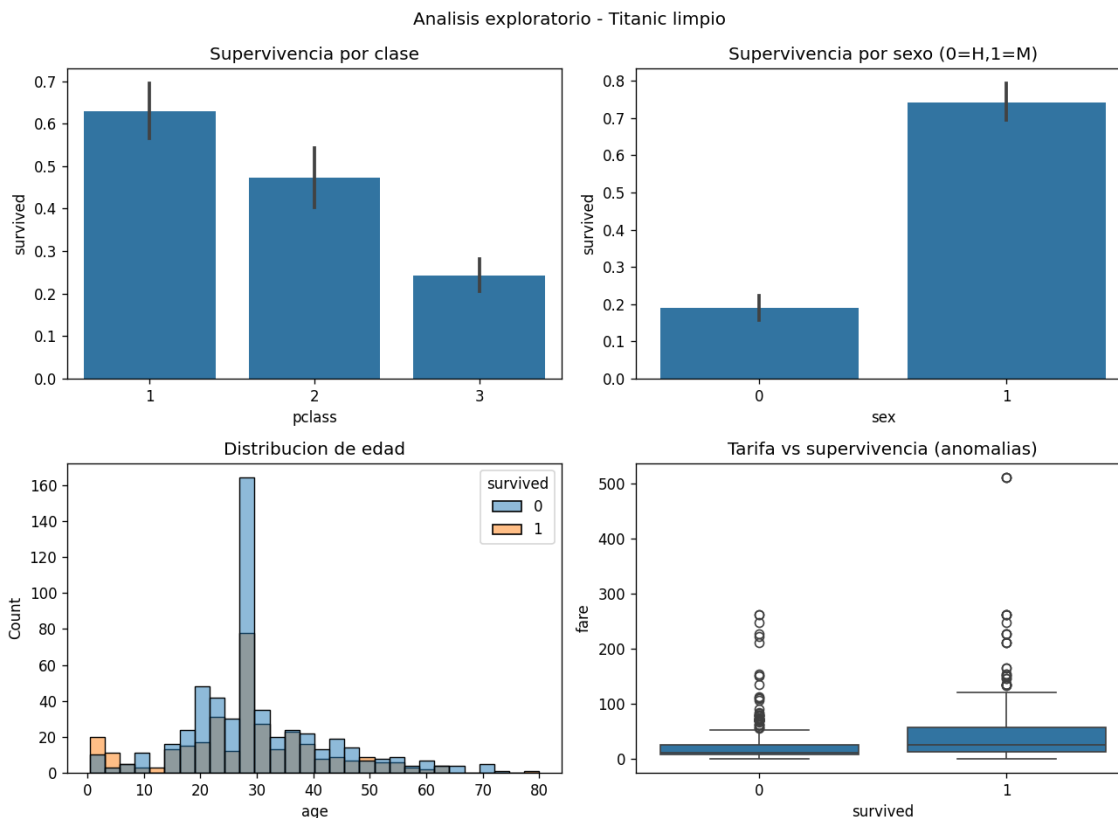
Figura 1. Patrones: la supervivencia aumenta en primera clase y es notablemente mayor en mujeres; el boxplot de tarifa muestra valores atípicos (anomalías).
