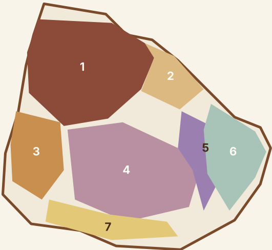
Esquema según la Carta Geológica 1:500.000 (Bossi y Ferrando, 2001).
