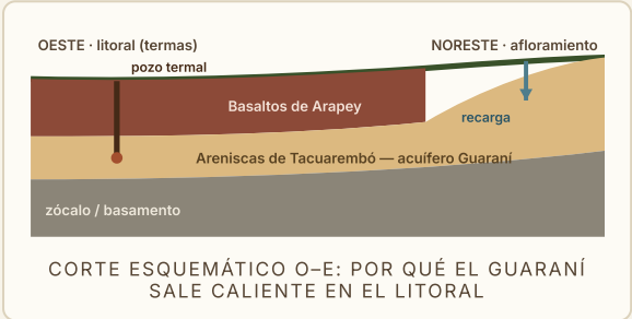
Esquema según cartas hidrogeológicas DINAMIGE (1986–2003).
