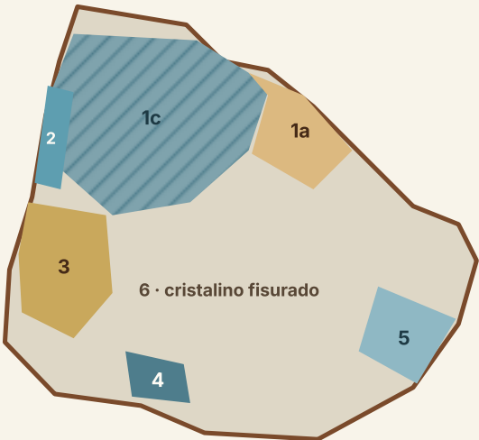
Esquema según cartas hidrogeológicas DINAMIGE (1986–2003).
