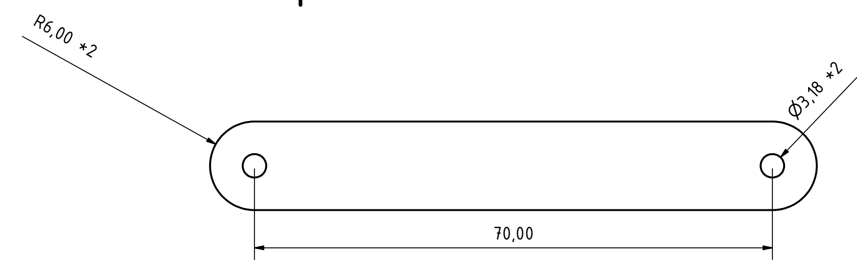
Barra 1.ipt Espesor: 3mm
