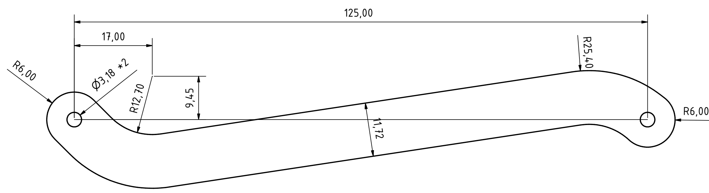
Barra 1.ipt Espesor: 3mm
