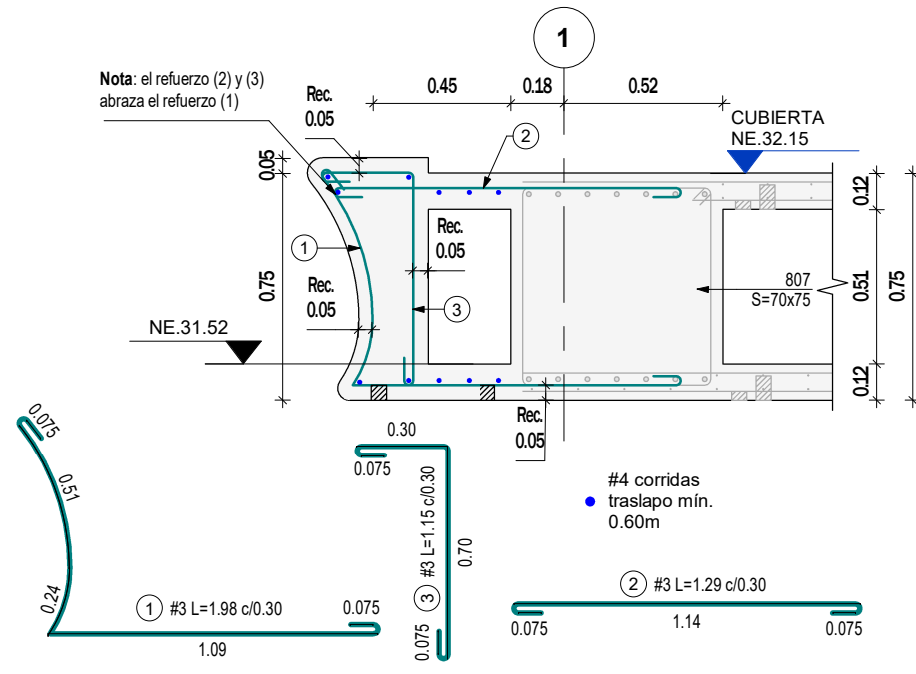
CORTE 4 - 4 Escala 1 : 25
