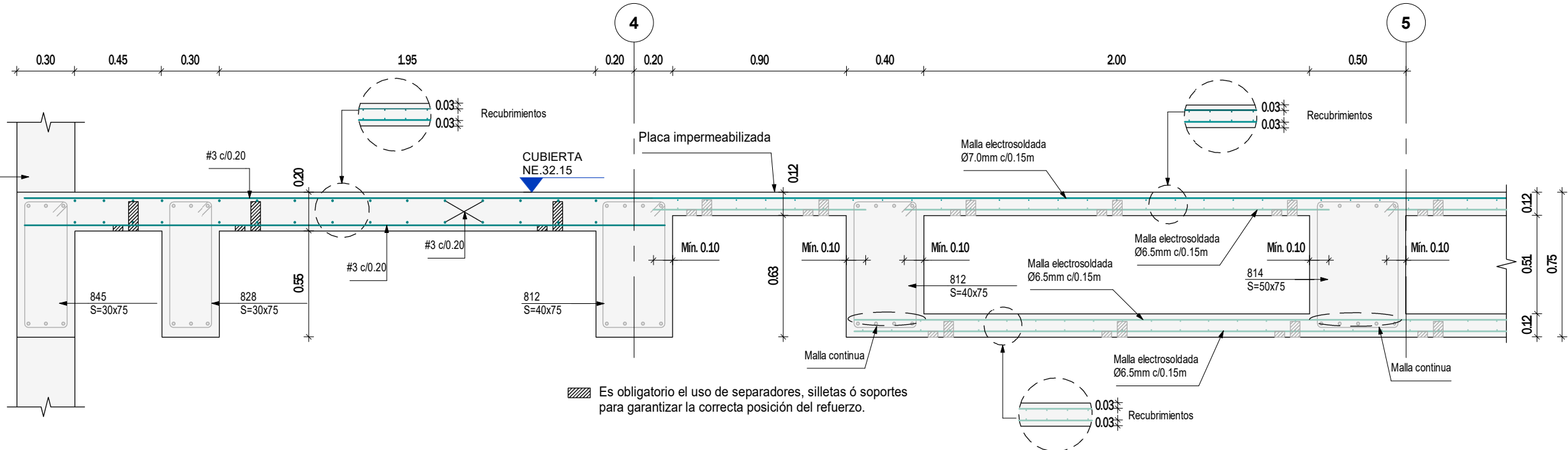
CORTE 3 - 3 Escala 1 : 25
