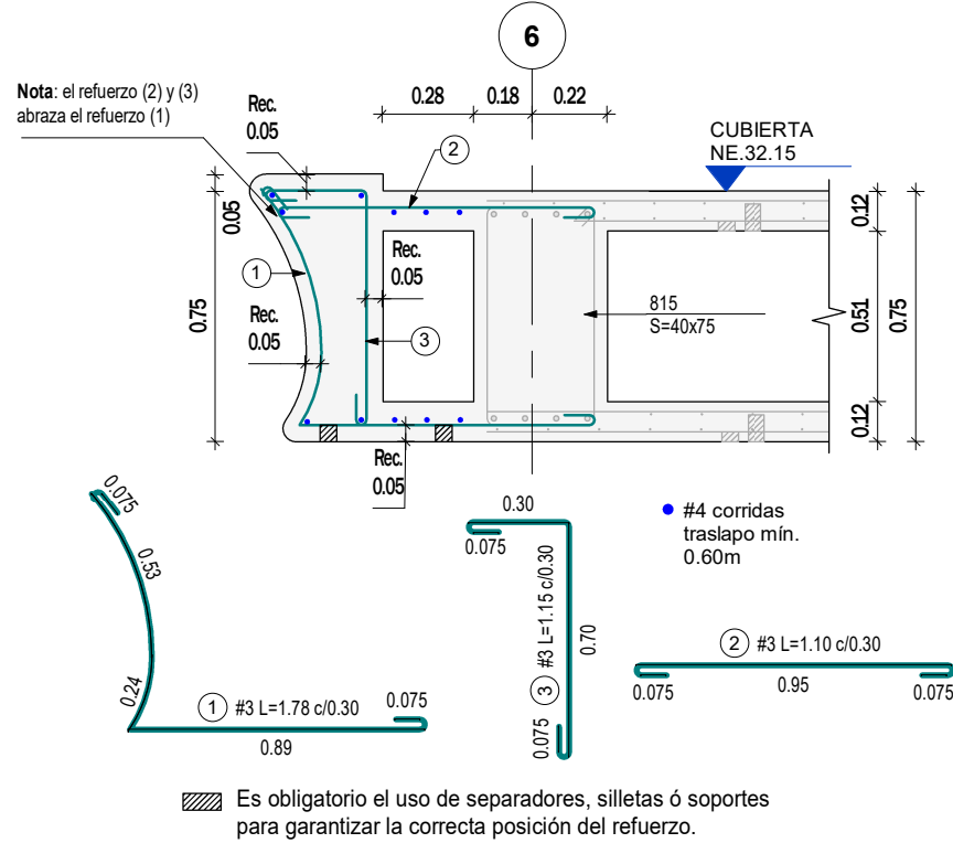
CORTE 5 - 5 Escala 1 : 25
