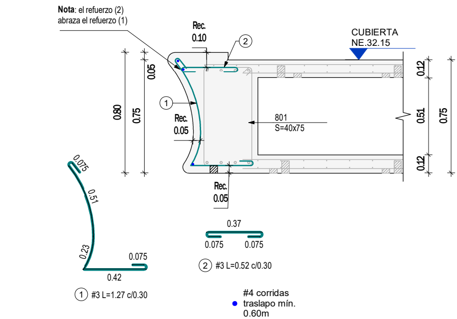
CORTE 1 - 1 Escala 1 : 25
