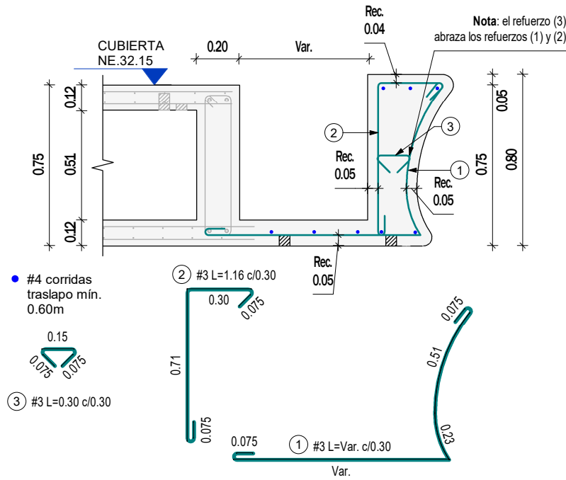
CORTE 2 - 2 Escala 1 : 25
