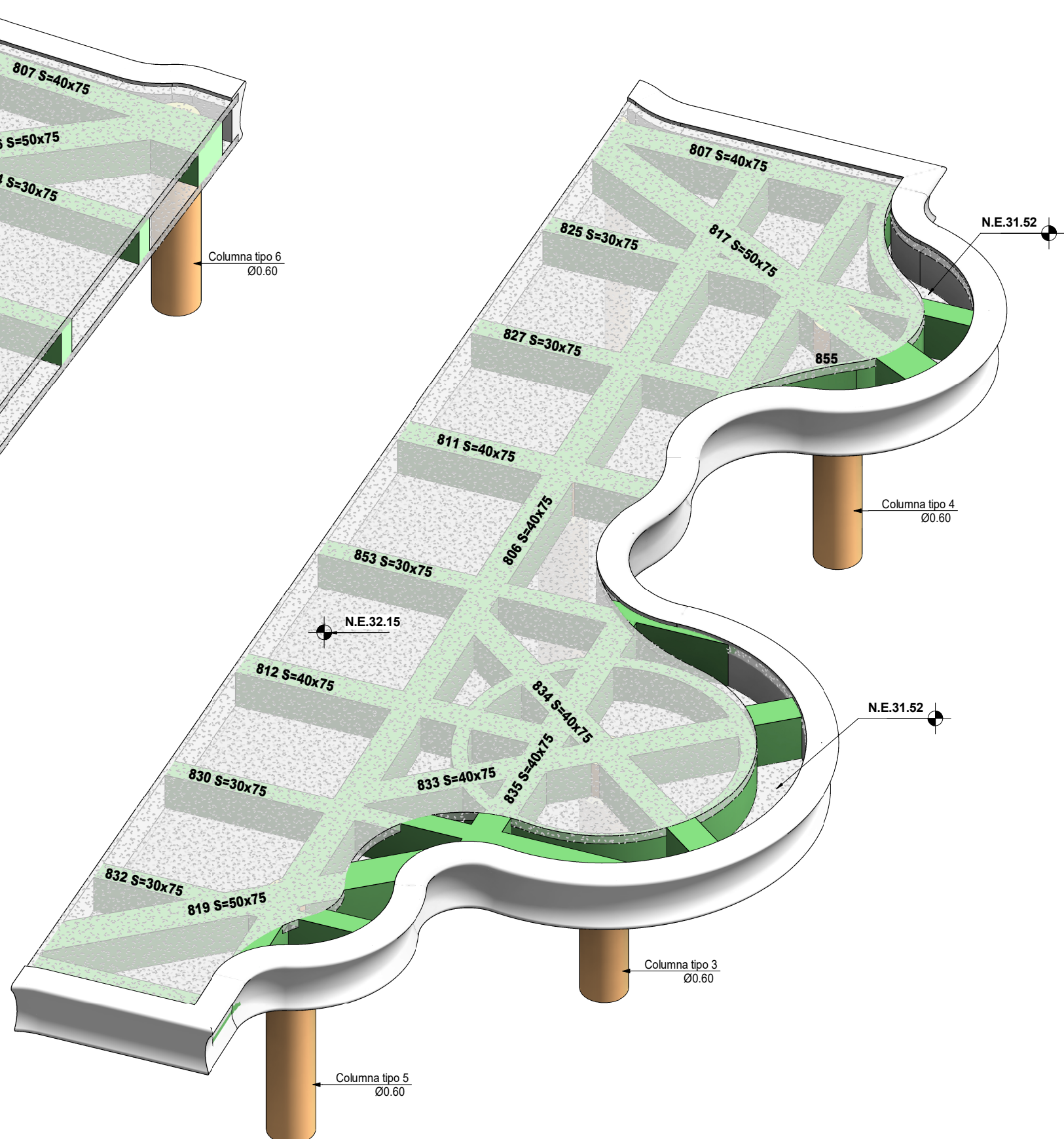
ESQUEMA 3D CUBIERTA DE BALCON COSTADO NORTE CUBIERTA Sin escala
