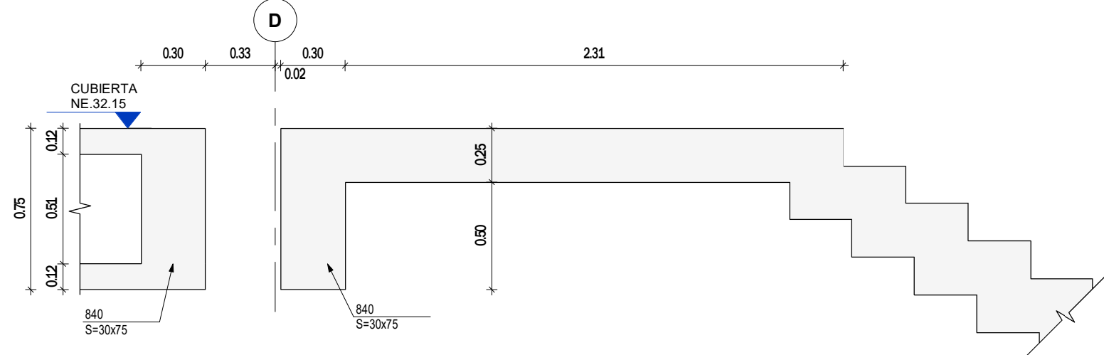
CORTE 6 - 6 Escala 1 : 25
