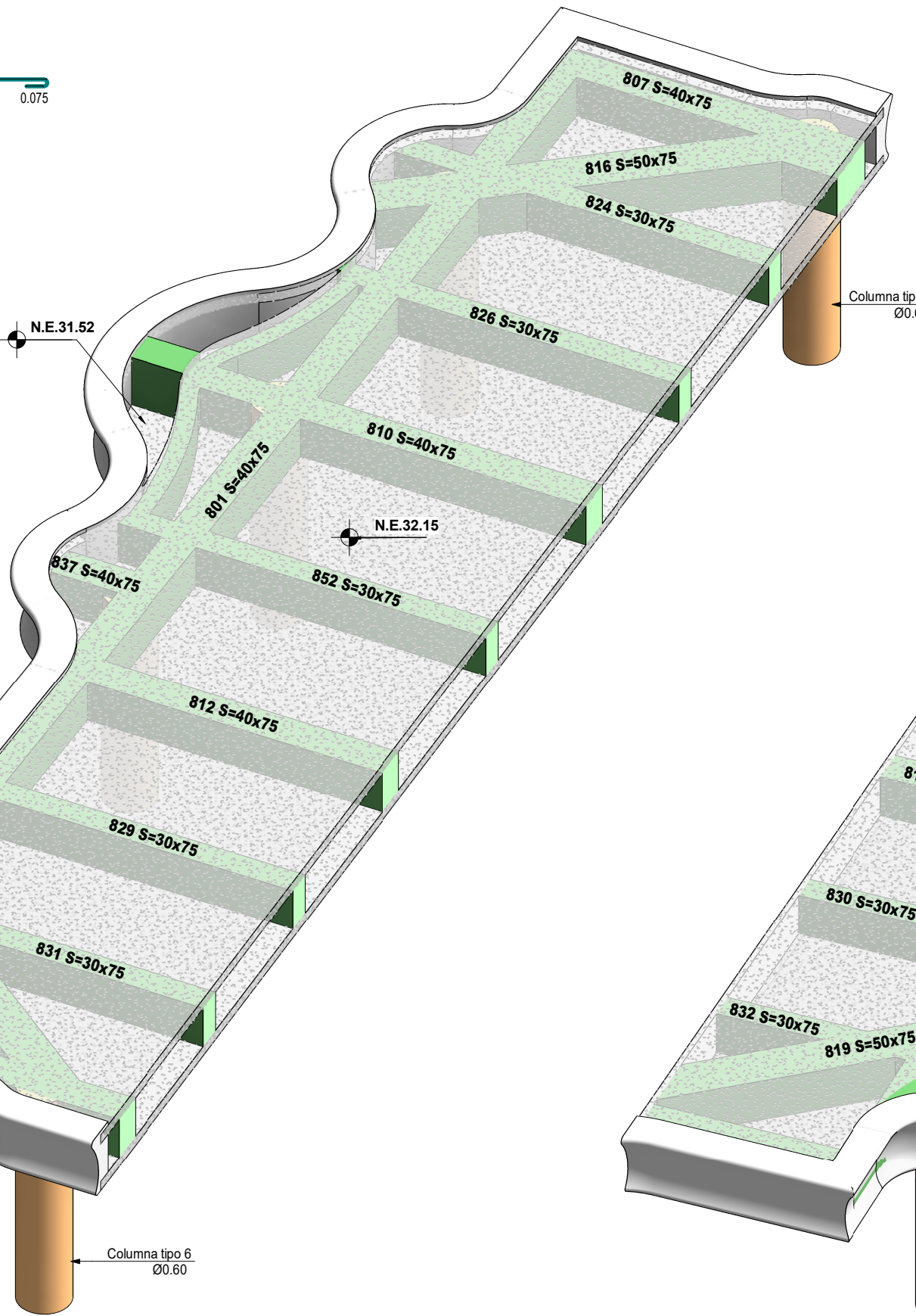
ESQUEMA 3D CUBIERTA DE BALCON COSTADO SUR CUBIERTA Sin escala
