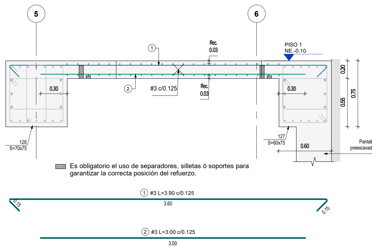
CORTE 1 - 1 Escala 1 : 25
