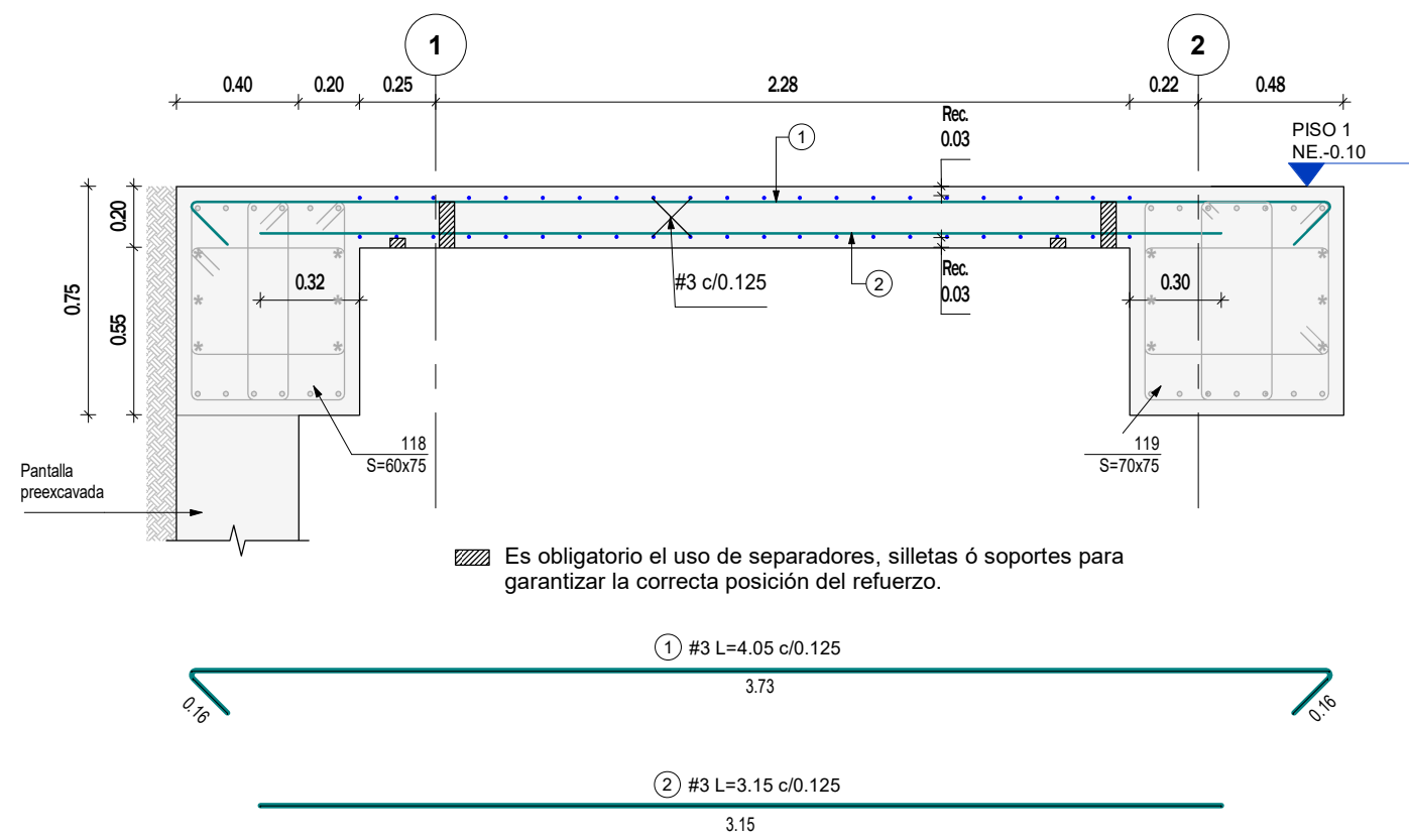
CORTE 1 - 1 Escala 1 : 25
