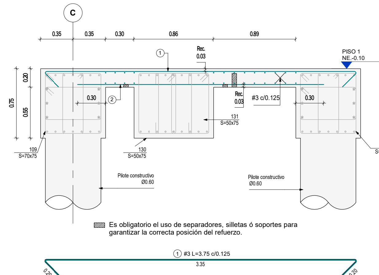
CORTE 4 - 4 Escala 1 : 25
