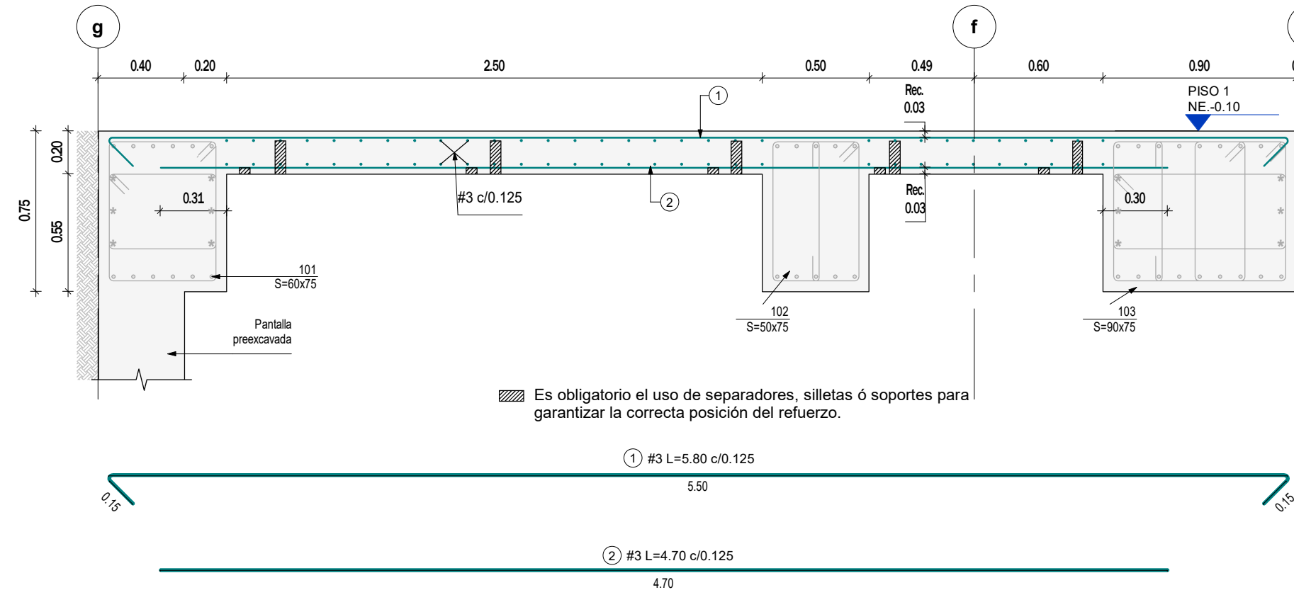
CORTE 2 - 2 Escala 1 : 25
