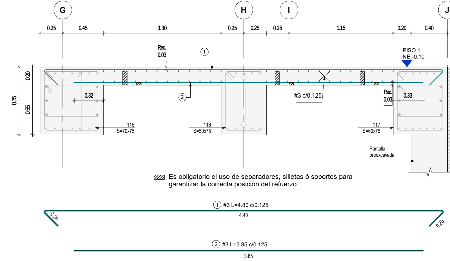
CORTE 2 - 2 Escala 1 : 25
