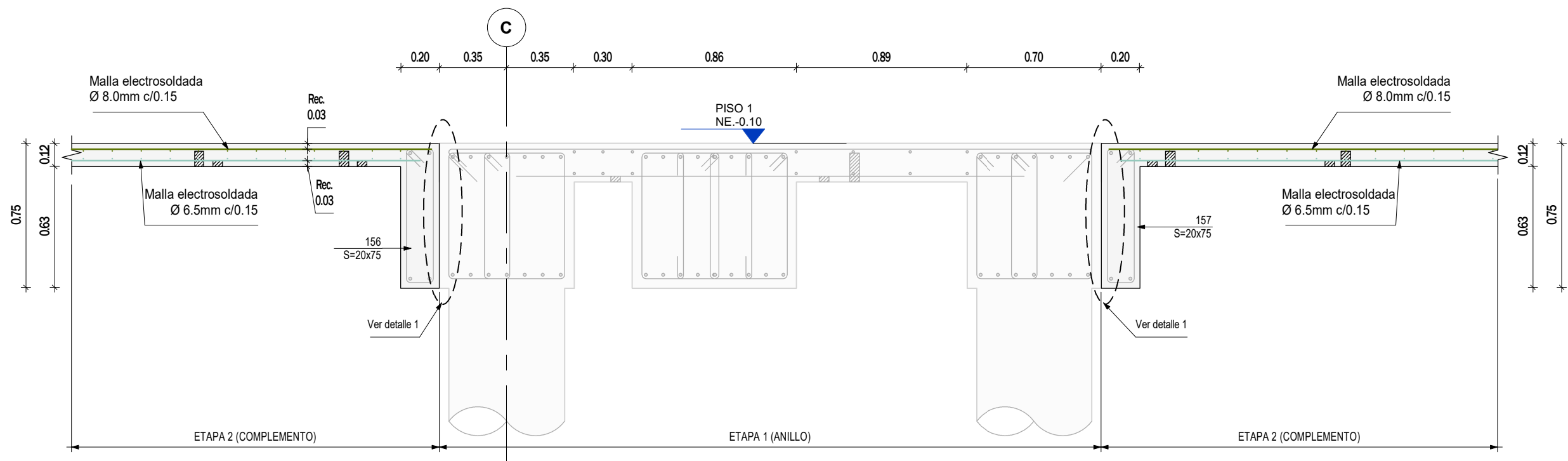
CORTE 2 - 2 Escala 1 : 25
