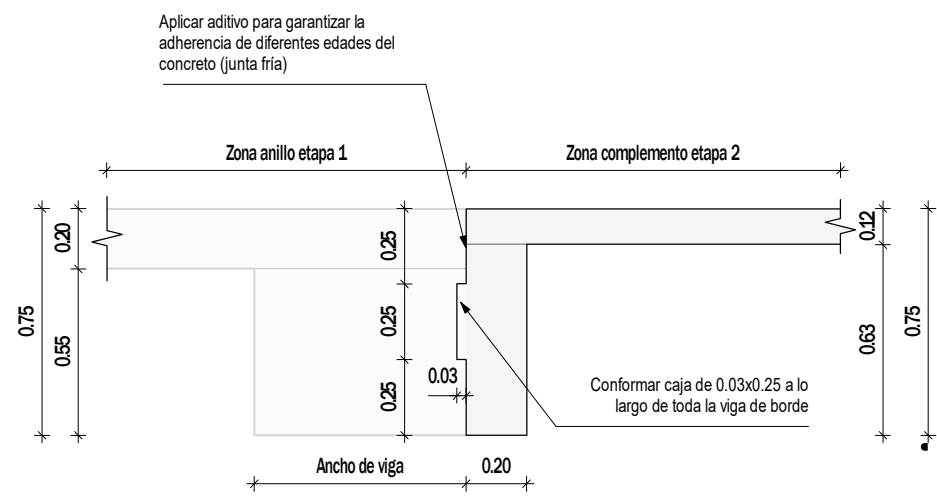
DETALLE 1 VINCULACIÓN DE VIGAS ETAPA 1 Y ETAPA 2 Escala 1 : 25
