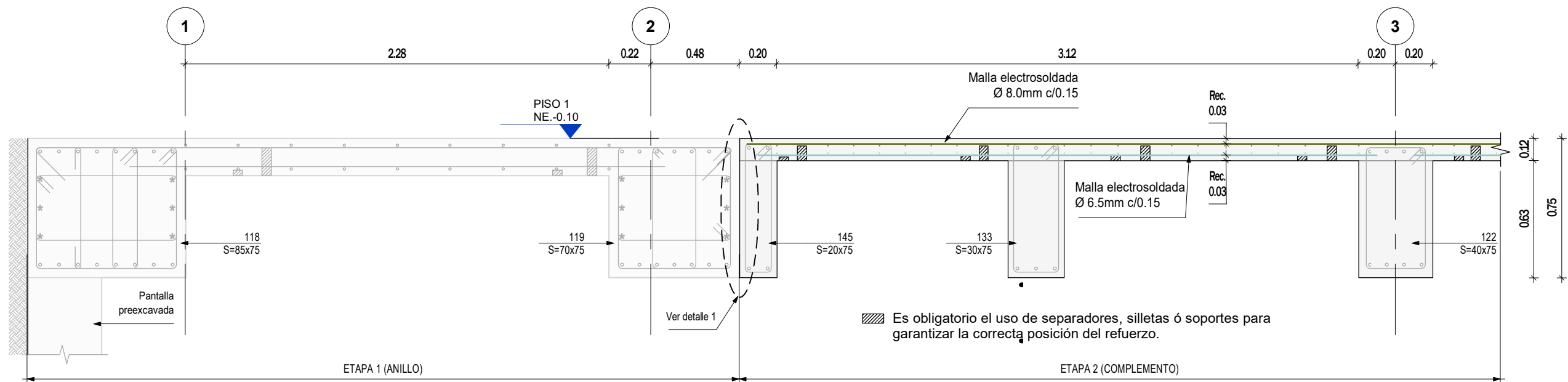
CORTE 1 - 1 Escala 1 : 25
