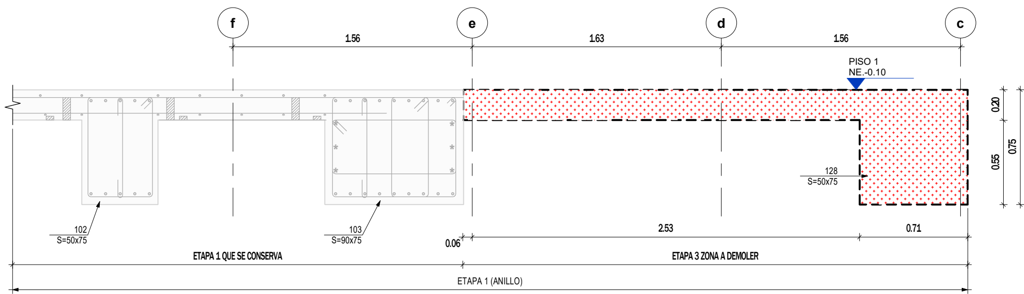
CORTE 1 - 1 Escala 1 : 25
