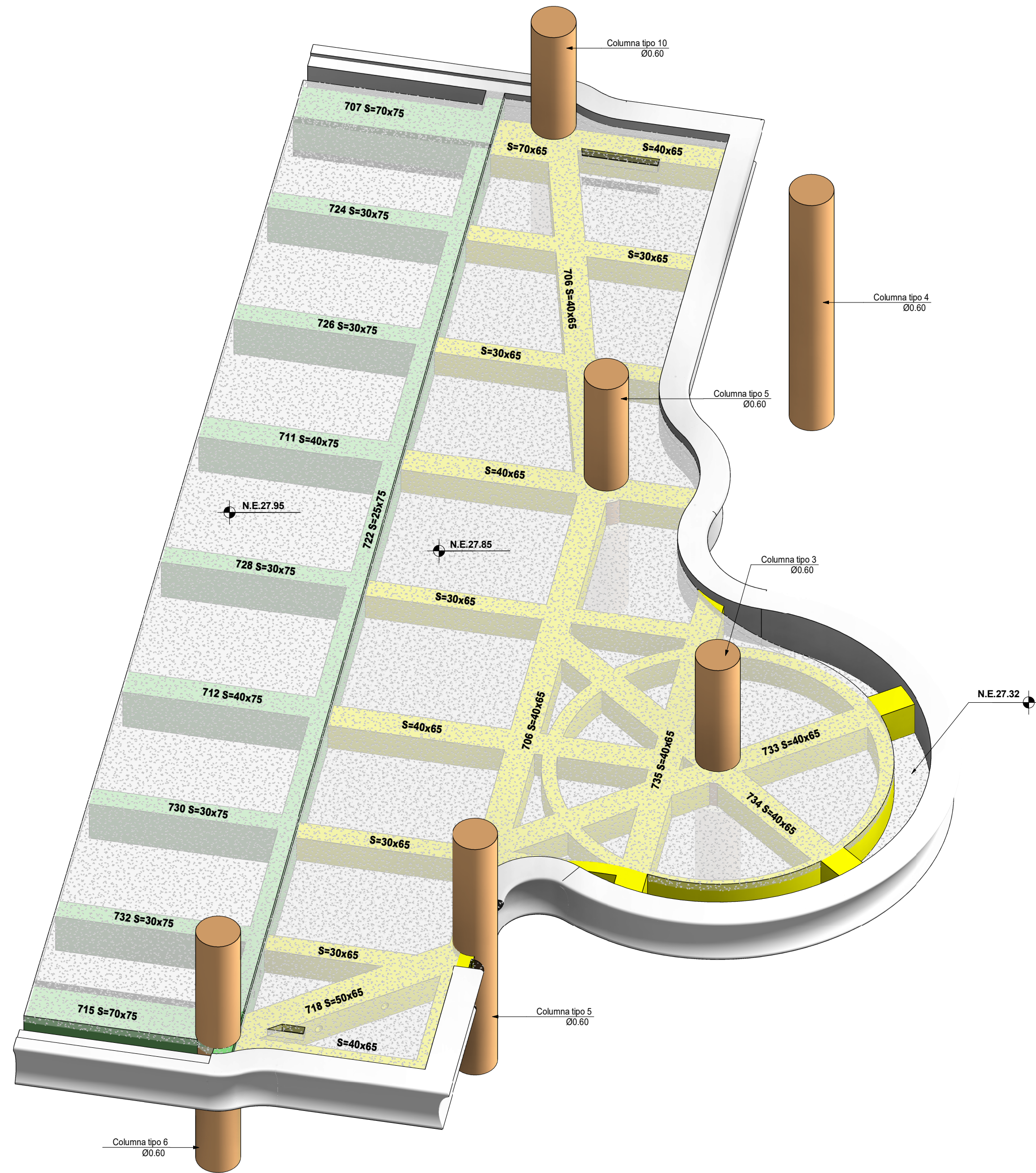
ESQUEMA 3D BALCON COSTADO NORTE PISO 7 Sin escala
