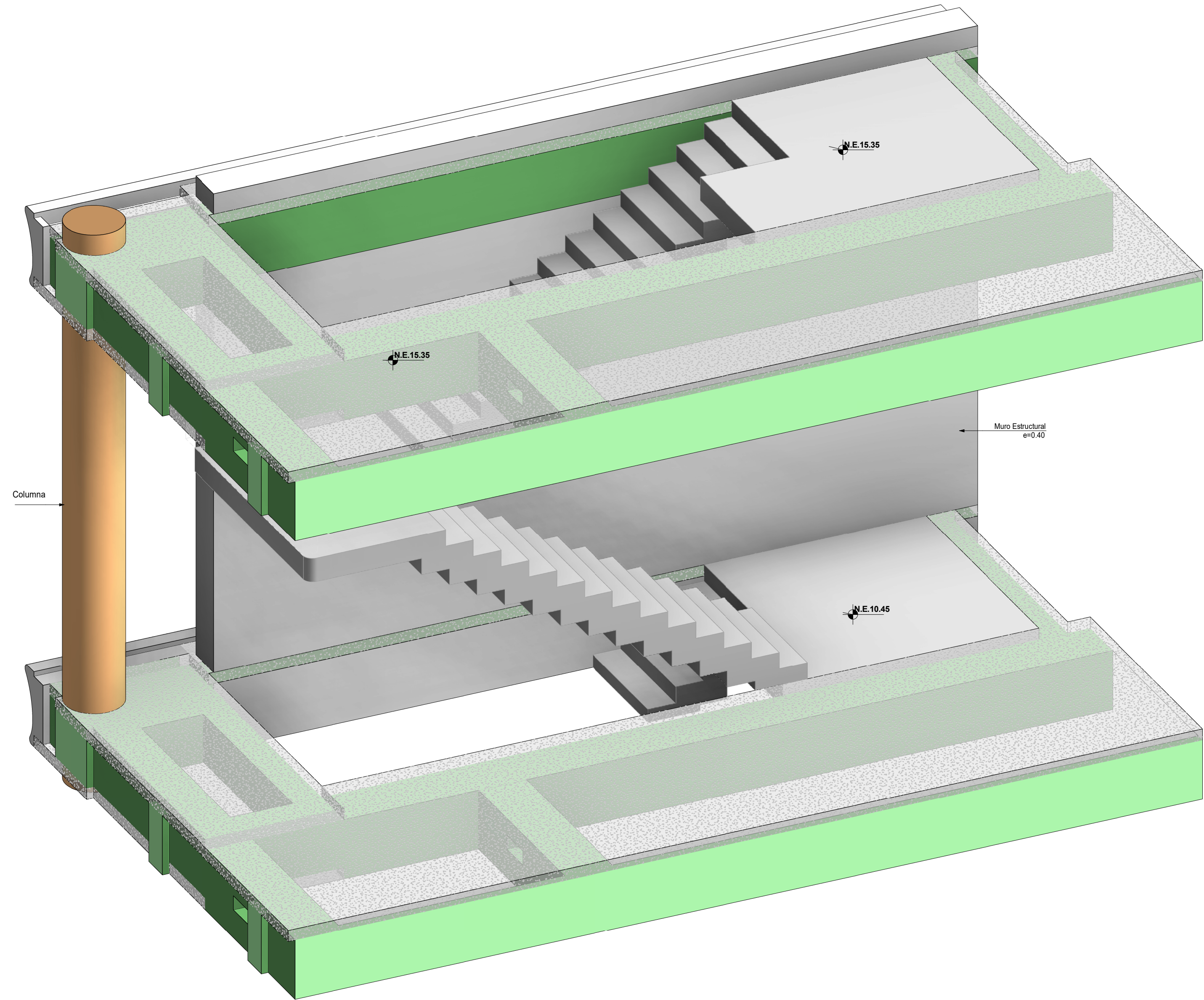
ESQUEMA 3D ESCALERA TIPO 2 PISO 3 A PISO 4 Sin escala
