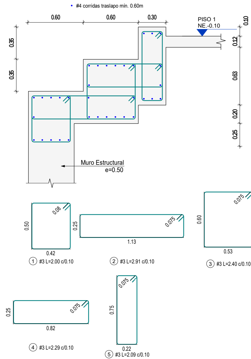
DETALLE 1 VIGAS CORONA ANFITEATRO Escala 1 : 25
