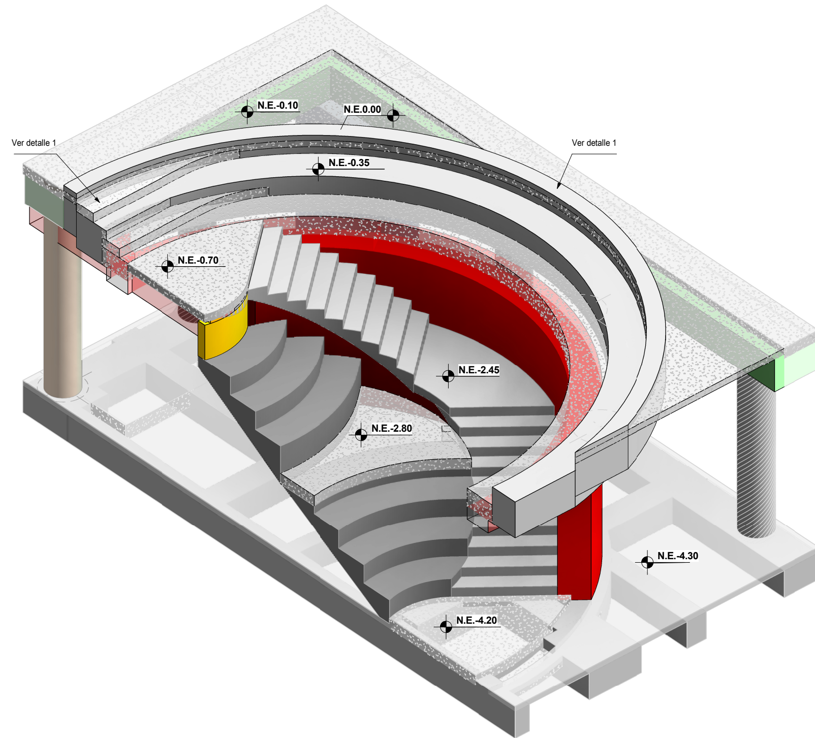
ESQUEMA 3D ESCALERA Y GRADERA ANFITEATRO Sin escala
