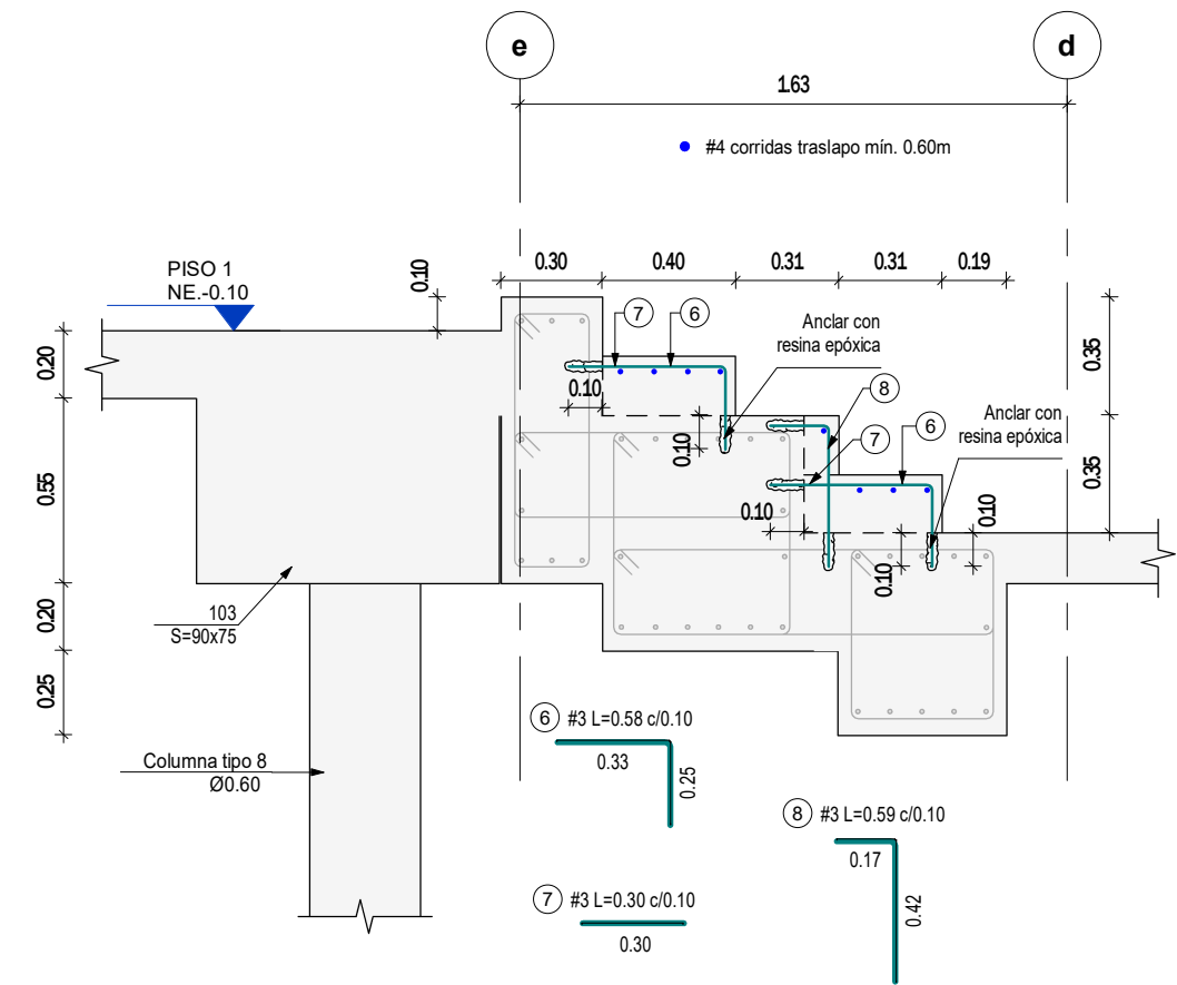
DETALLE 2 VIGAS CORONA ANFITEATRO Escala 1 : 25
