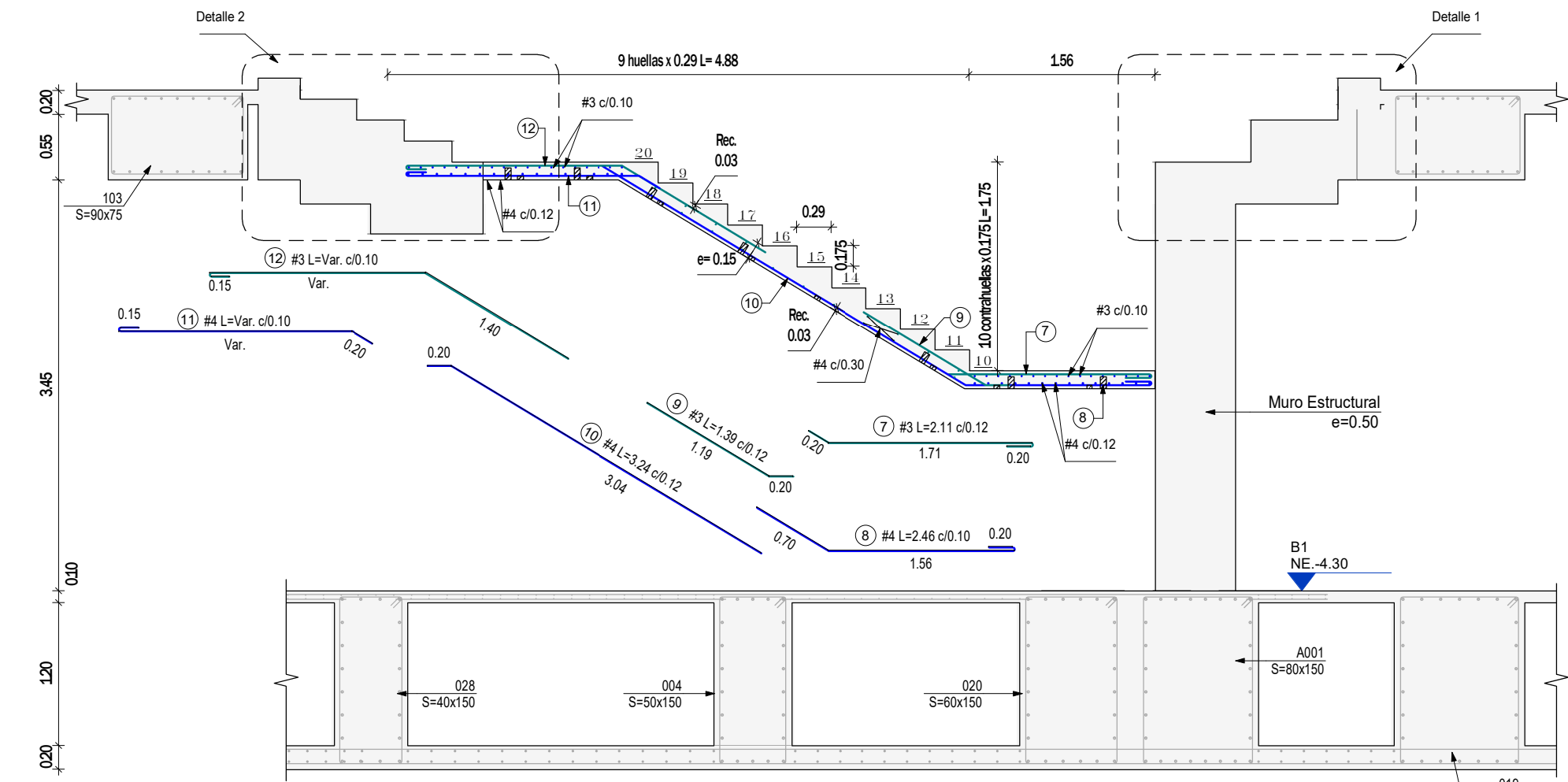
CORTE A3 Escala 1 : 50
