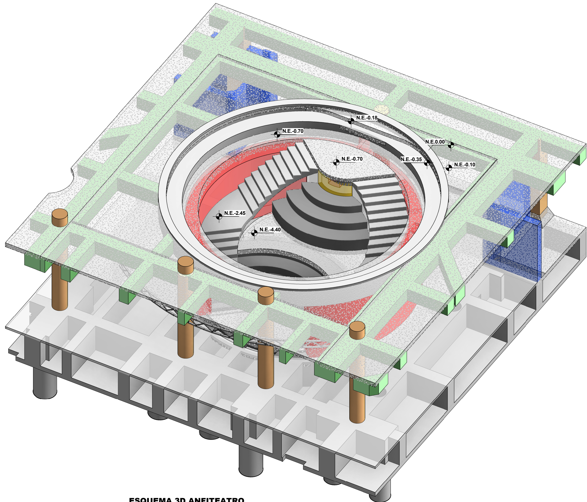
ESQUEMA 3D ANFITEATRO Sin escala
