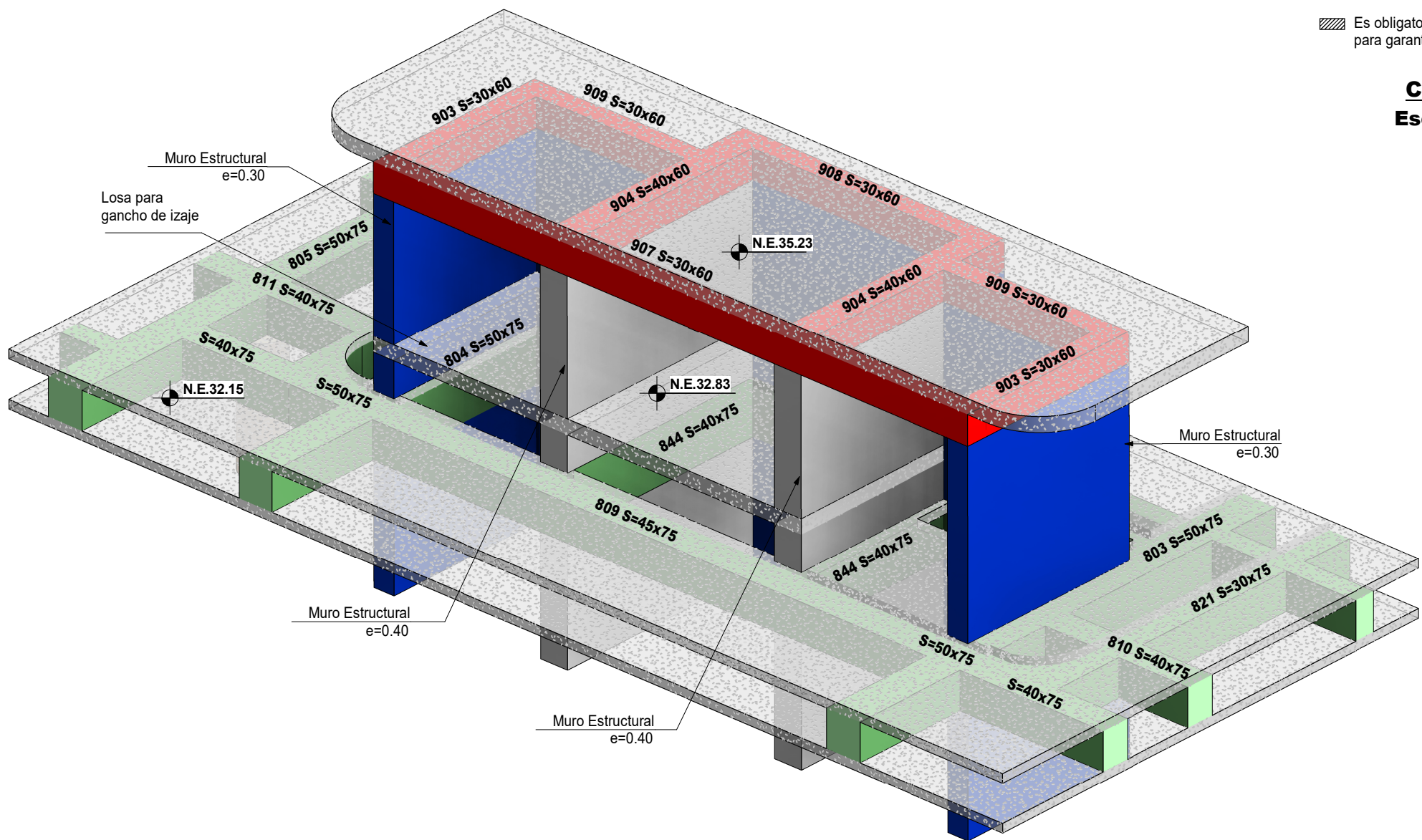
ESQUEMA 3D CUBIERTA ASCENSORES Sin escala
