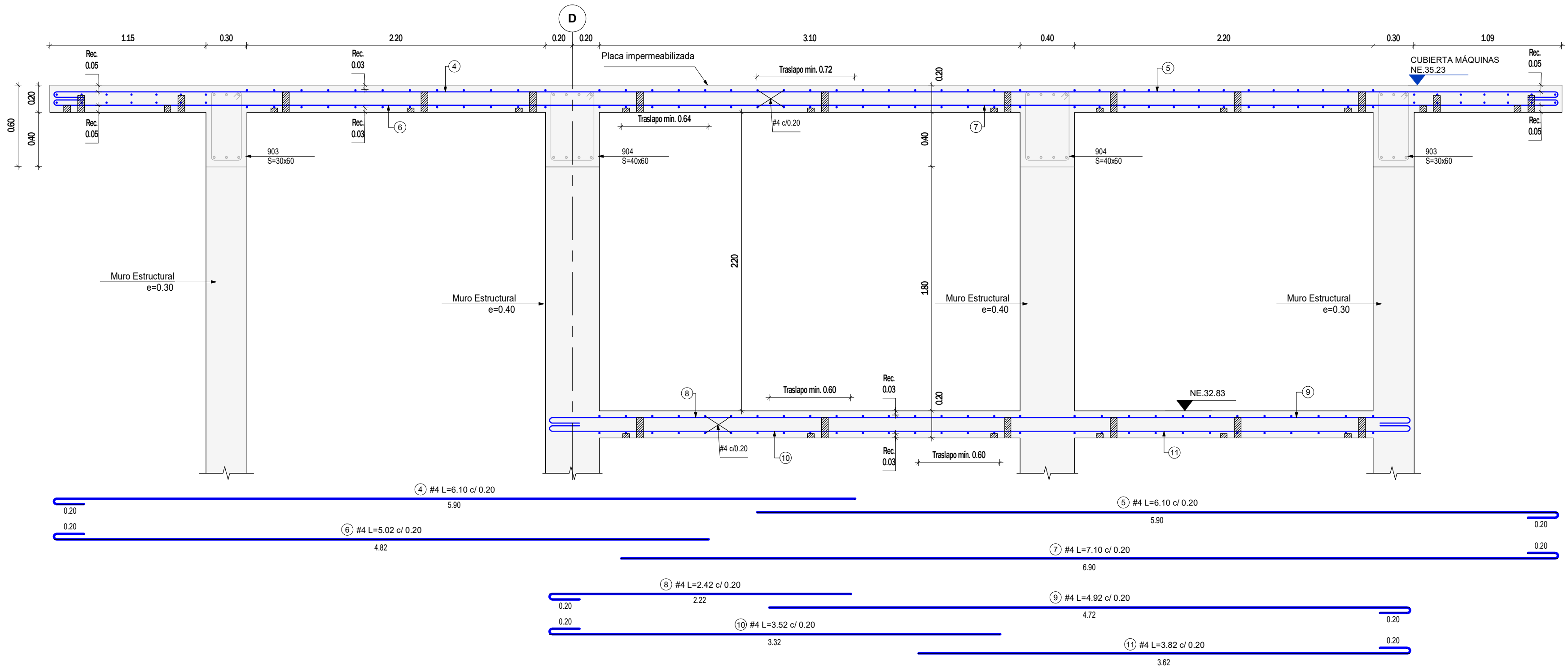
CORTE 2 - 2 Escala 1 : 25
