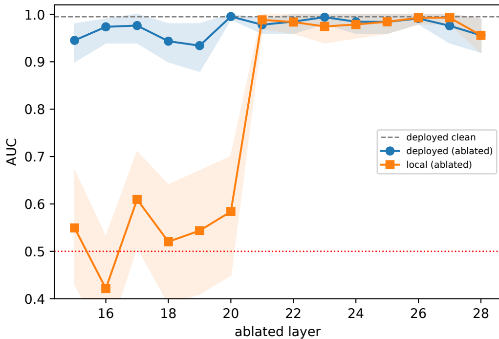
Qwen-3B
