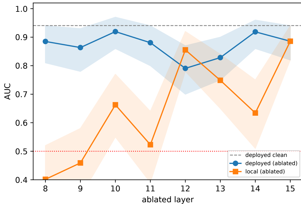
Gemma-2b
