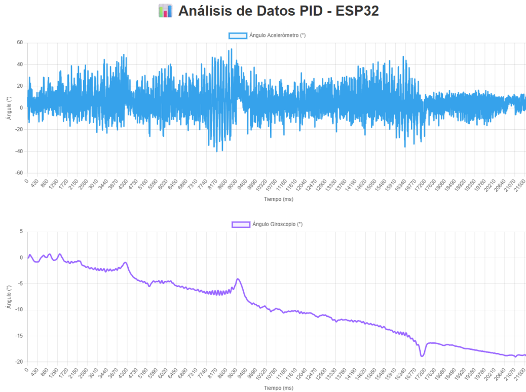
Figura 7.34: Señales de acelerómetro y giroscopio en función del tiempo (ms). Donde muestra cada sensor durante la operación del sistema.
