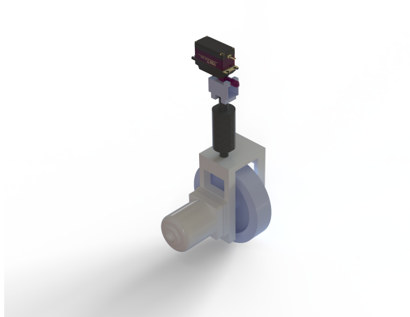
Figura 8.5: Detalle del diseño del volante en SolidWorks
