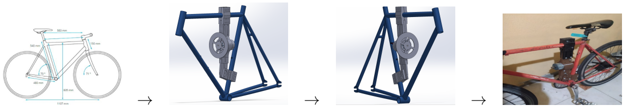
Figura 7.2: Secuencia del proceso de diseño del primer prototipo de volante de inercia (Diseño 3D e implementación)
