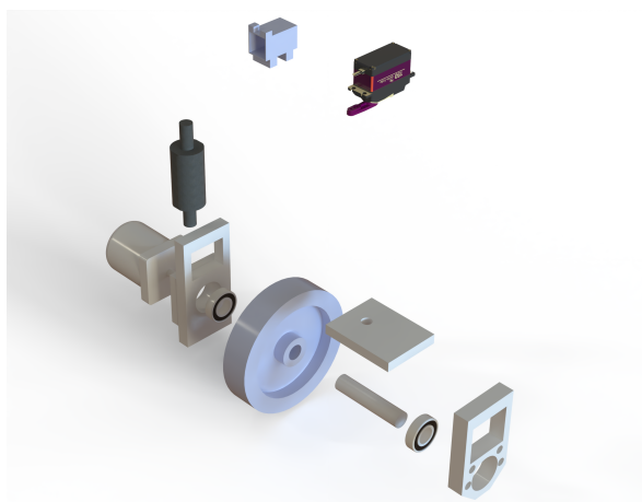
Figura 8.6: Despiece y vista explosionada del volante
