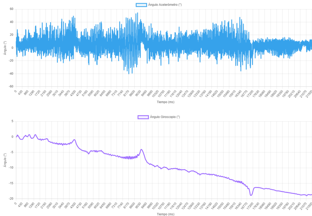
Figura 8.10: Señales de acelerómetro y giroscopio en función del tiempo (ms). Donde muestra cada sensor durante la operación del sistema.
