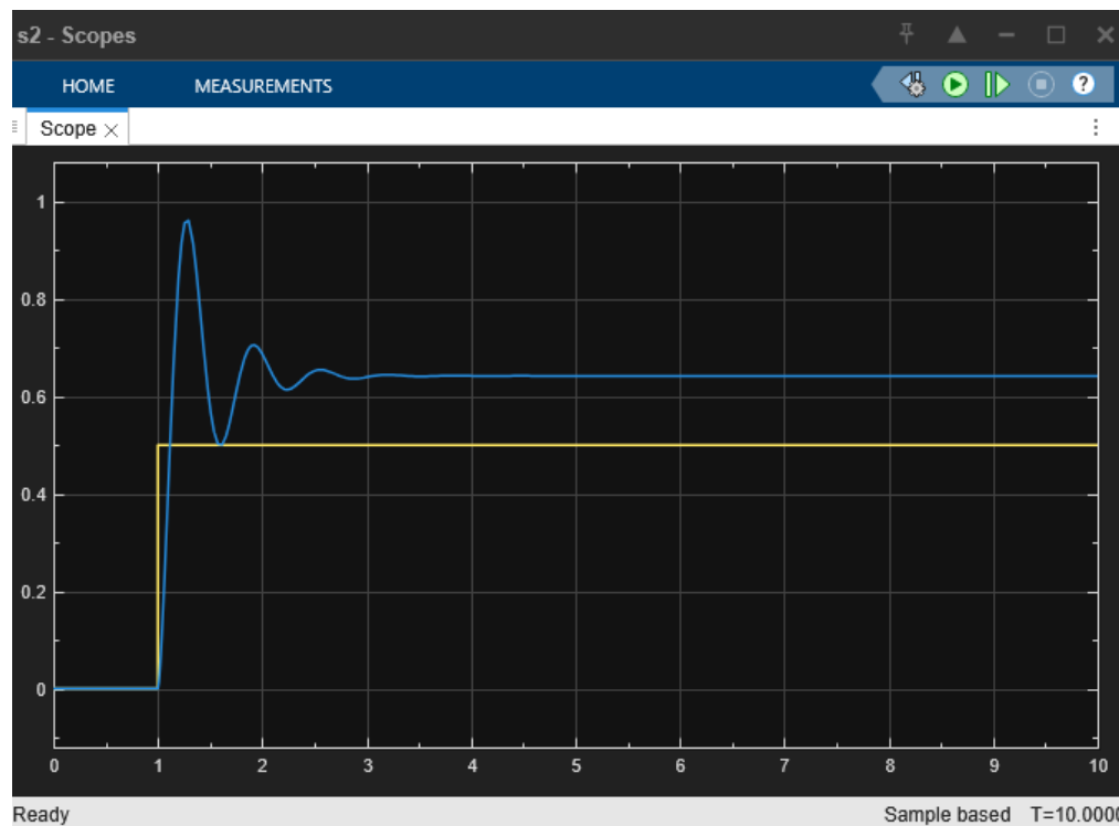
Figura 8.9: Respuesta del sistema con controlador PID ante perturbación inicial
