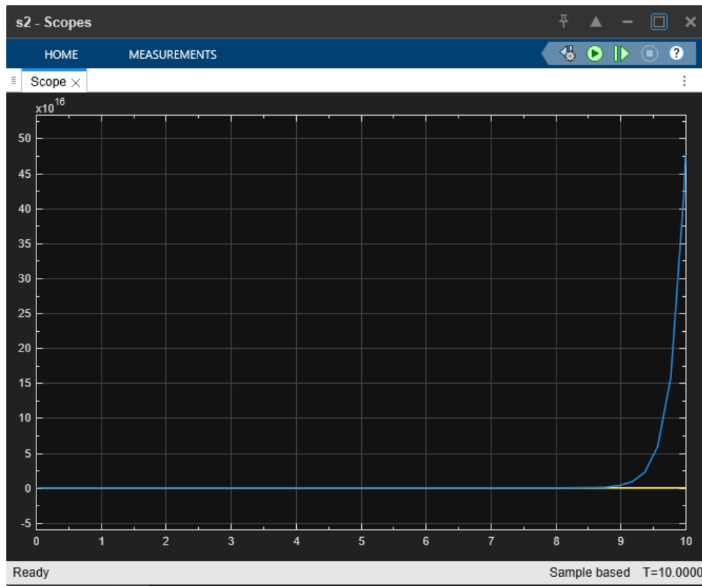
Figura 8.7: Respuesta del sistema a lazo abierto ante una entrada escalón de 0.5 rad
