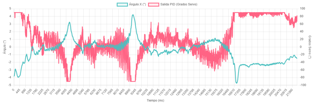
Figura 8.13: Comparación temporal entre el filtro complementario (medición del ángulo de inclinación) y la salida del controlador PID (comando al servomotor). Se observa la relación de fase y la capacidad del controlador para estabilizar el sistema.
