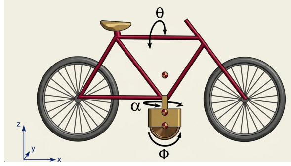
Figura 7.1: Diagrama de Cuerpo Libre para el análisis de inercia del sistema
