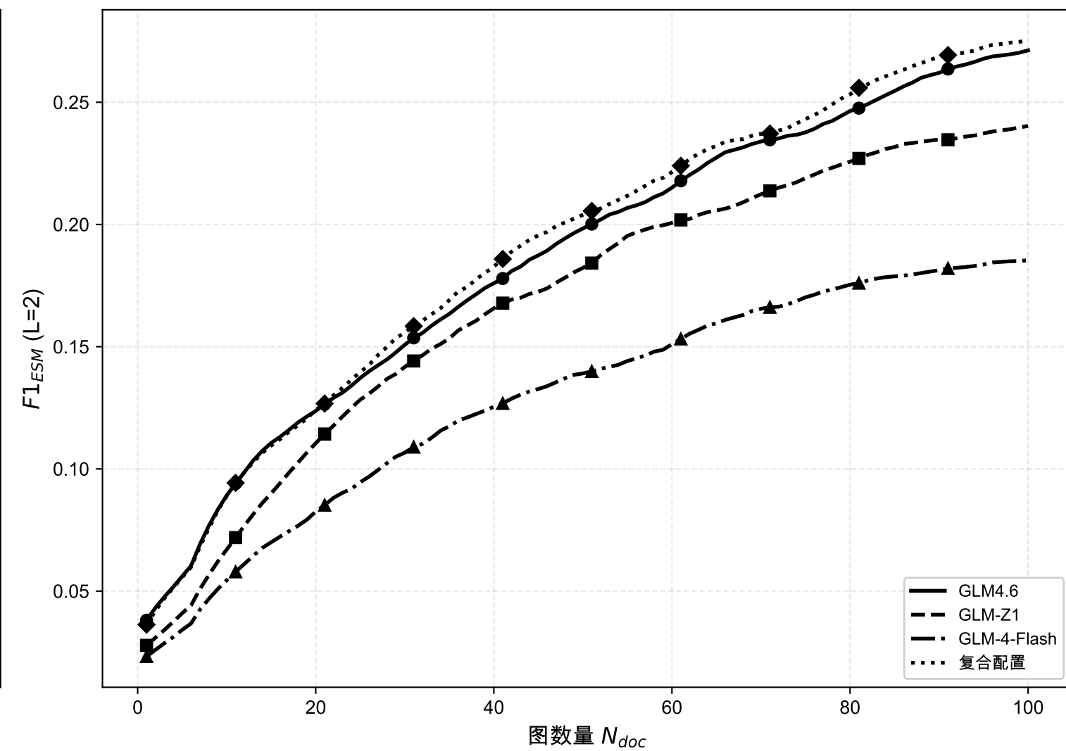
(d) 性能边际效益
