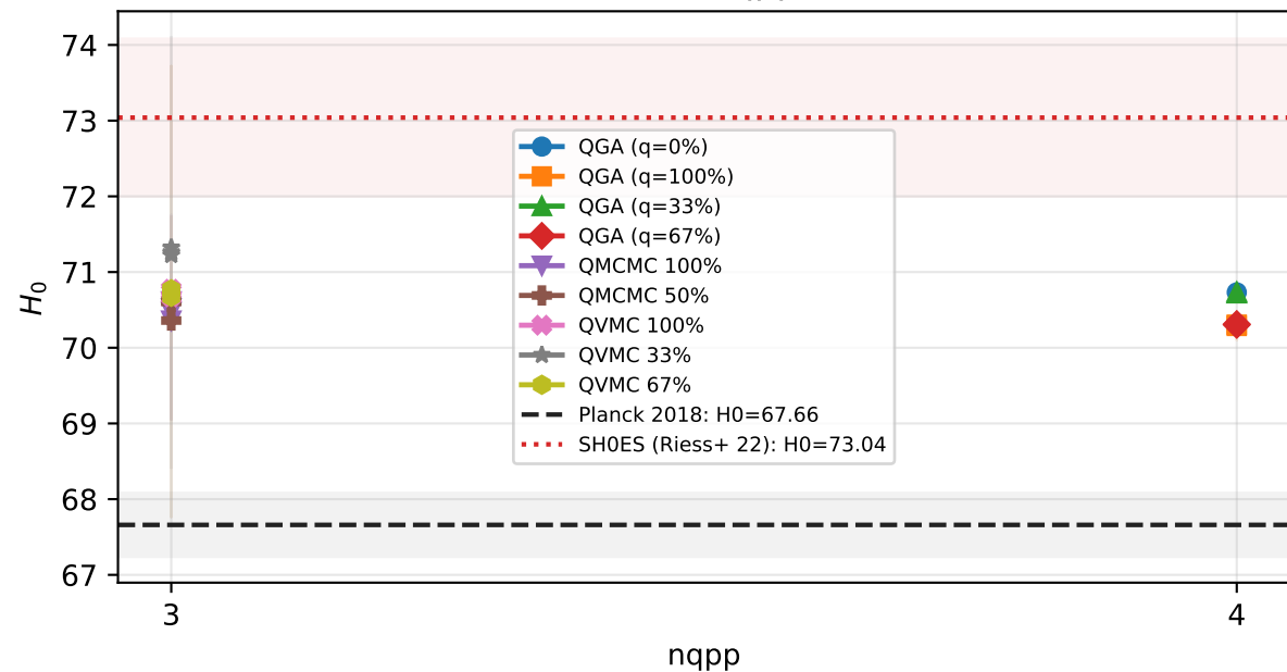
H_0 vs nqpp
