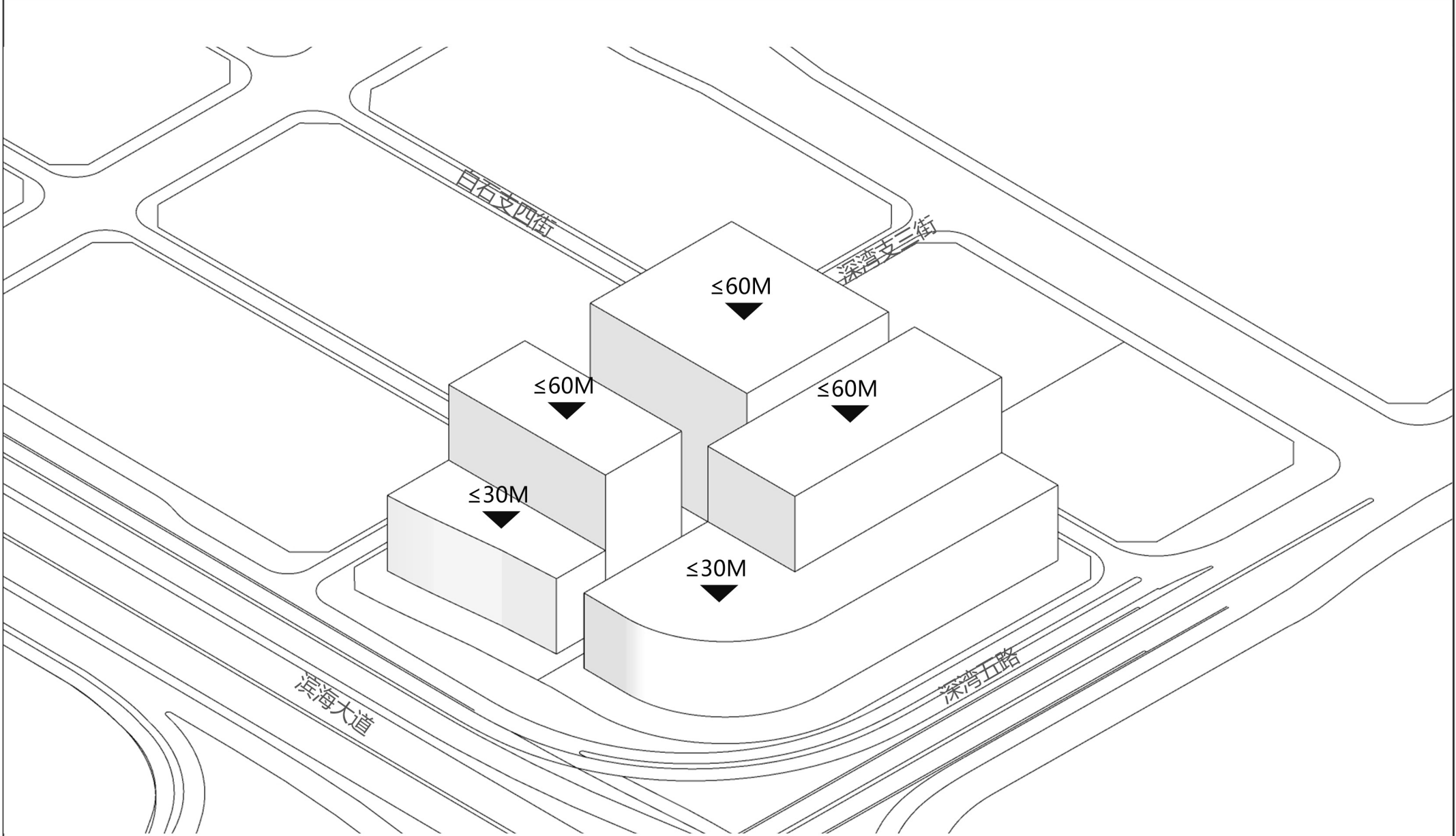
建筑高度控制图
