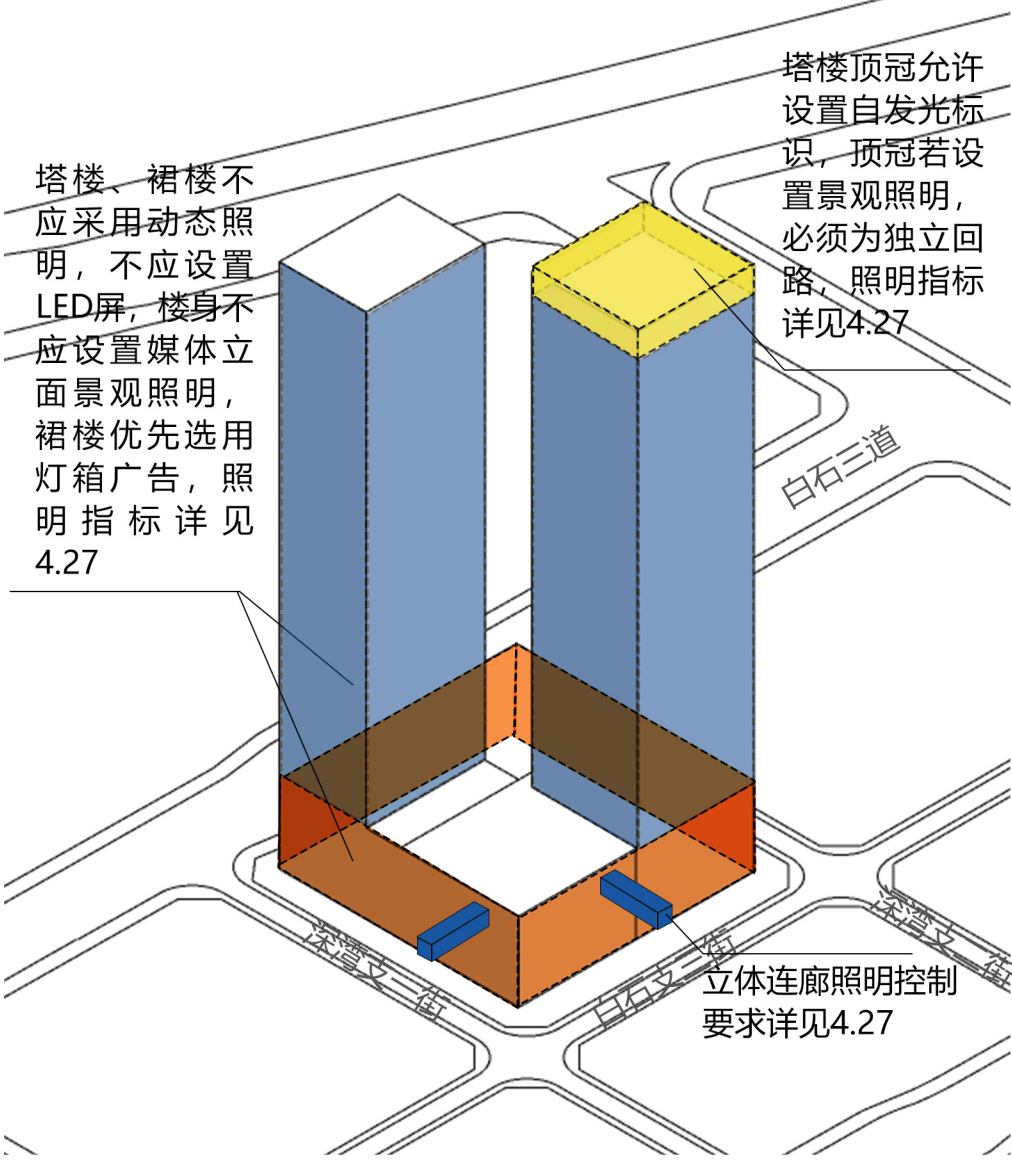
立体照明控制图
