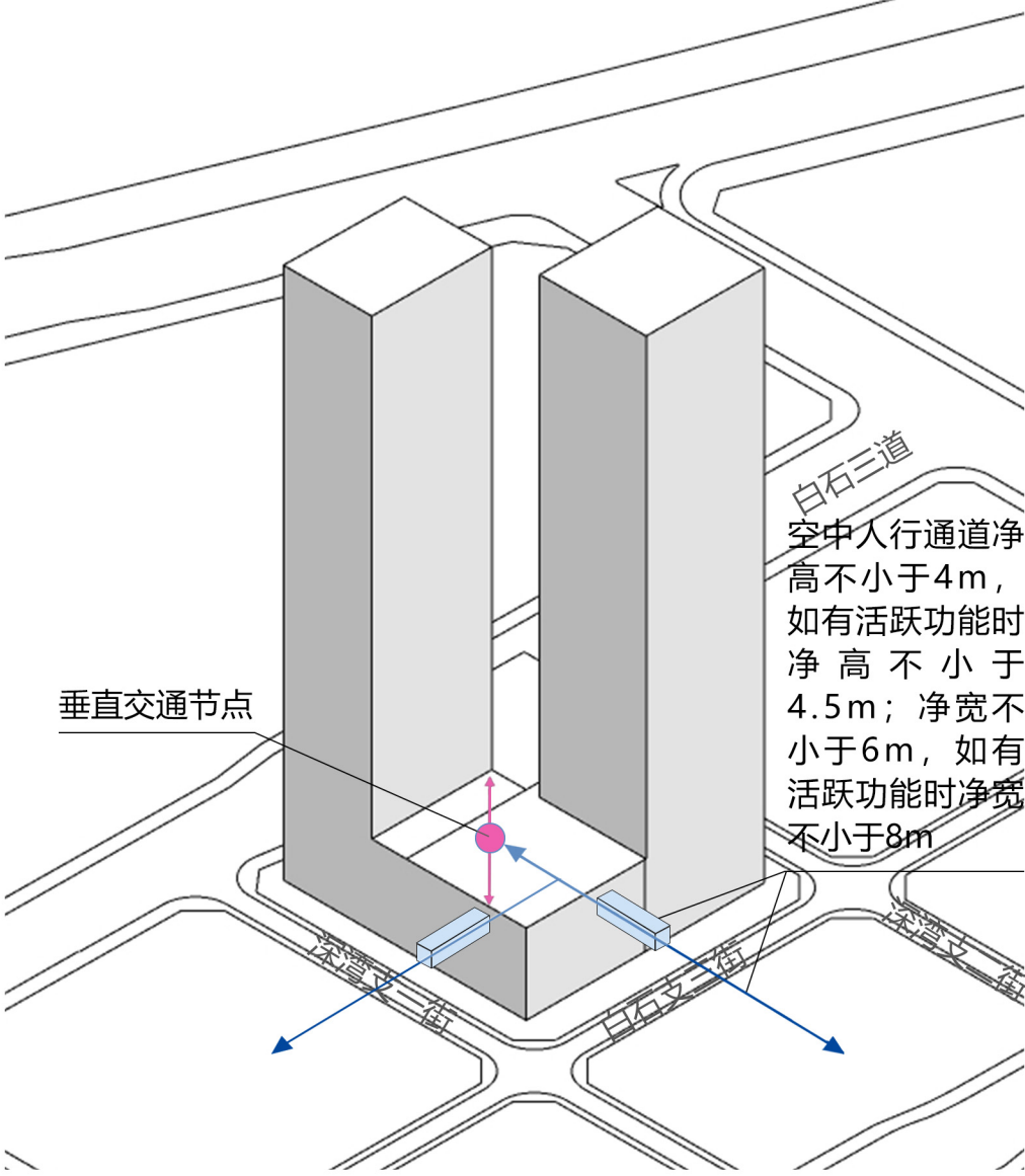
空中人行通道/垂直交通节点控制图
