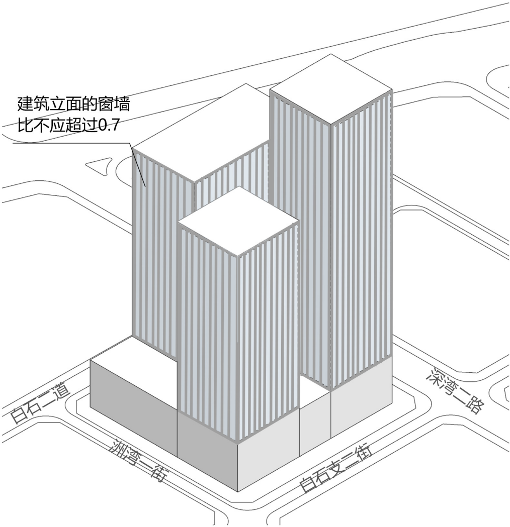
建筑立面控制图
