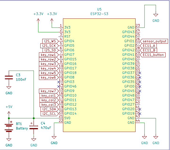
MCU
