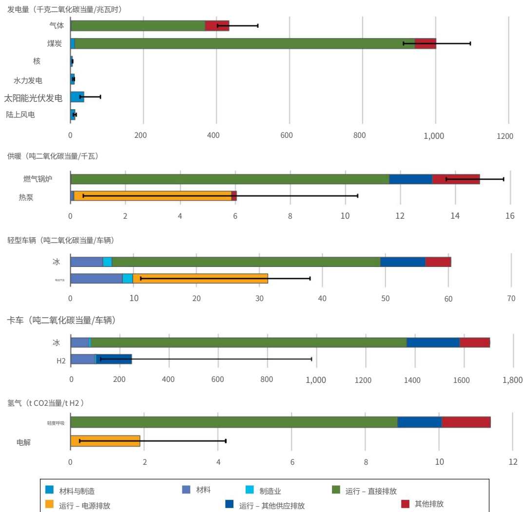
图表 30:部分能源技术的排放量
