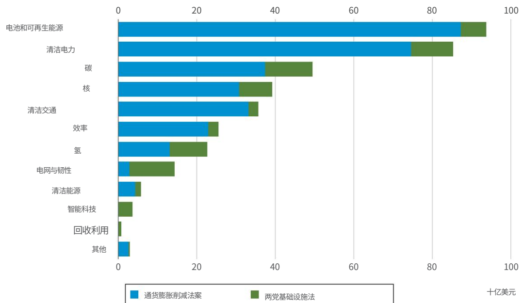
图表 14:按主题和来源划分的能源资金
