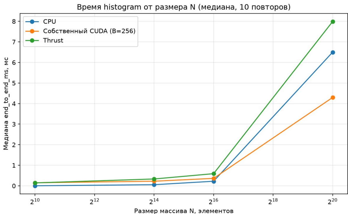
Рисунок 1 - Медиана end_to_end_ms от размера N
