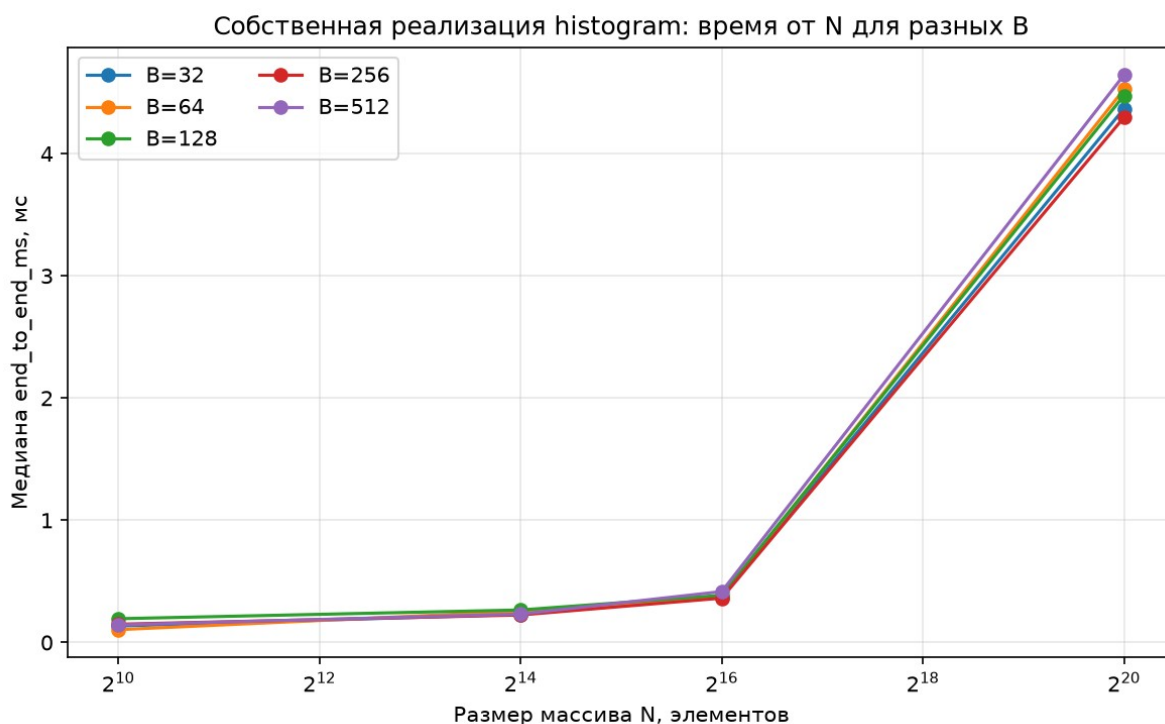
Рисунок 3 - Собственная реализация: end_to_end_ms от N для разных B
