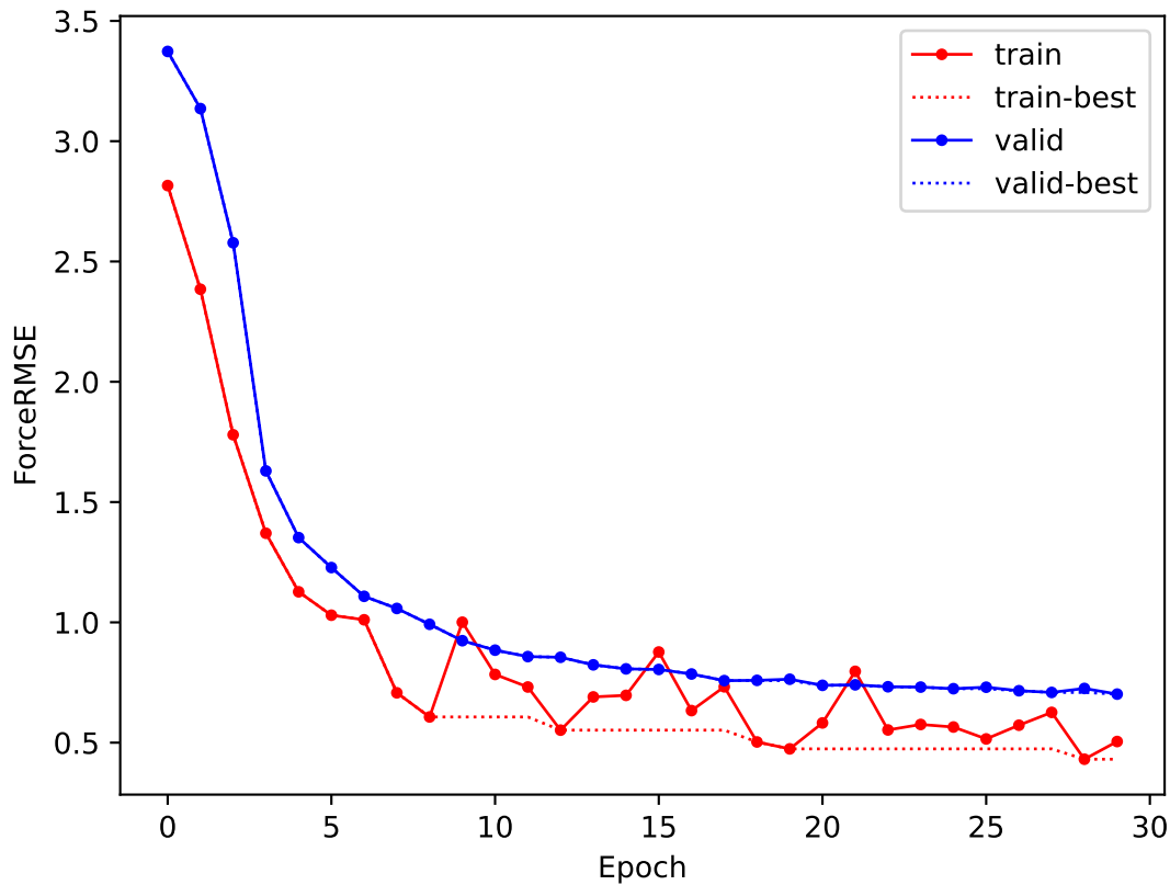
ForceRMSE
