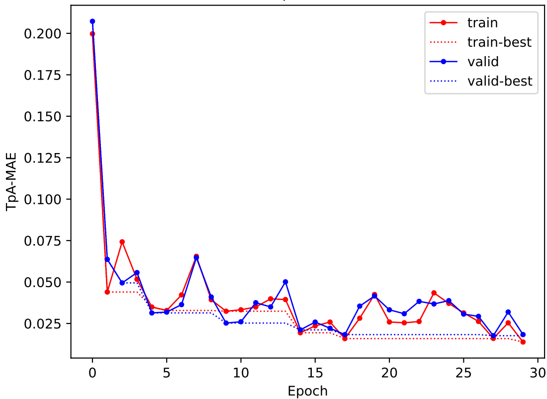
TpA-MAE
