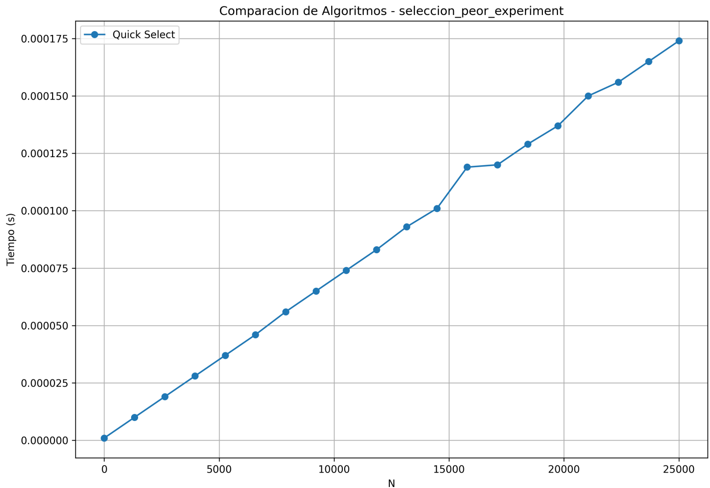
Figura 8. Quick Select: peor caso (pivote ultimo en arreglo ordenado).
