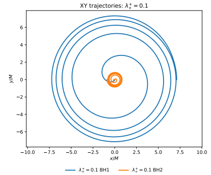
(d) q = 8 : orbital trajectories.
