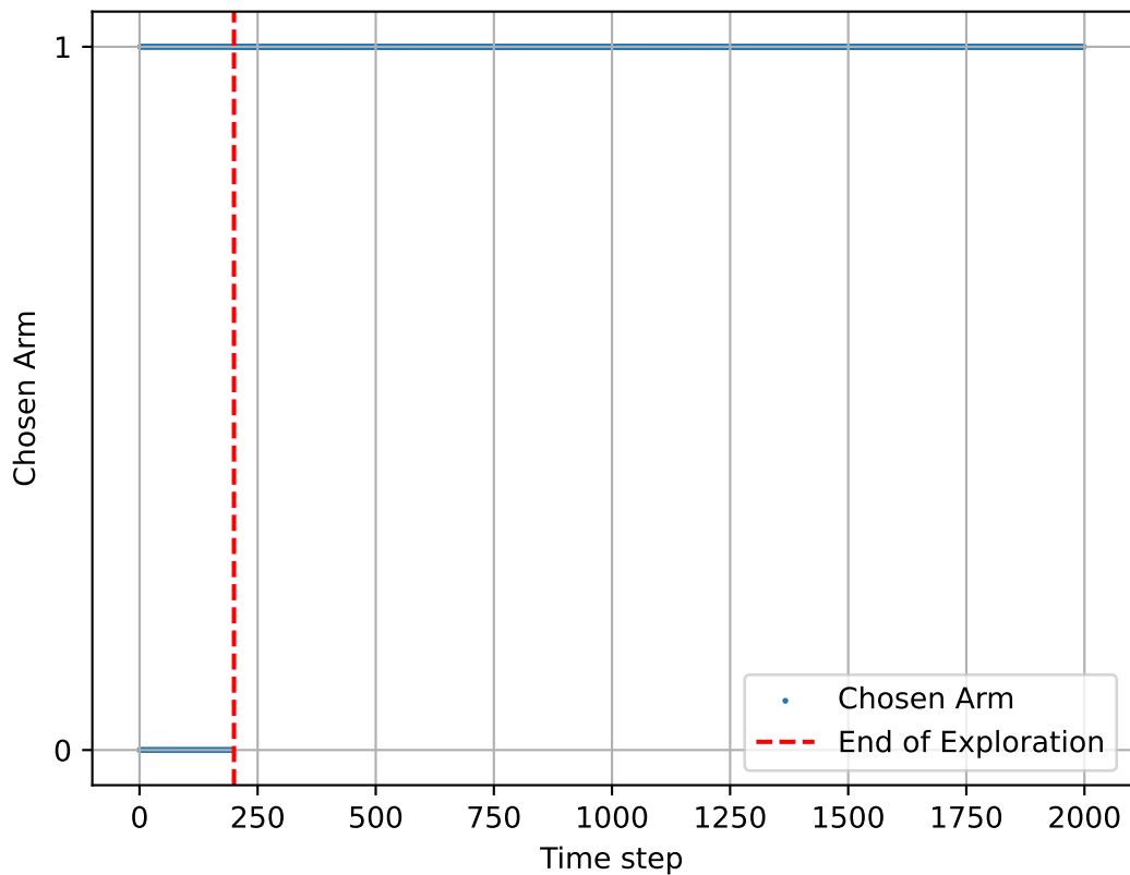
Chosen Arm over Time (ETC)
