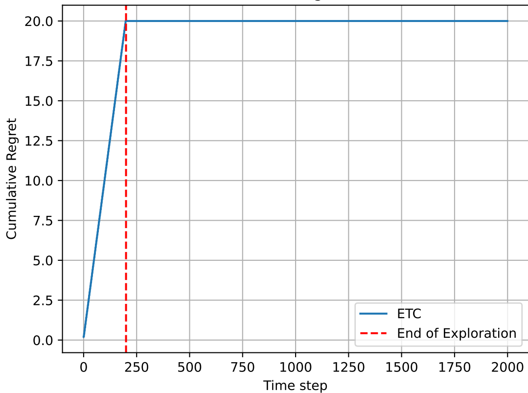
Cumulative Regret (ETC)
