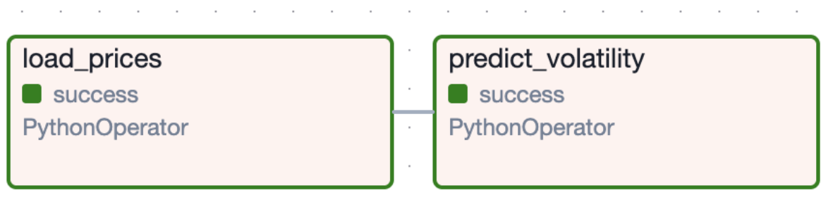
Рисунок 2.3 — Структура основного DAG-a Apache Airflow.
