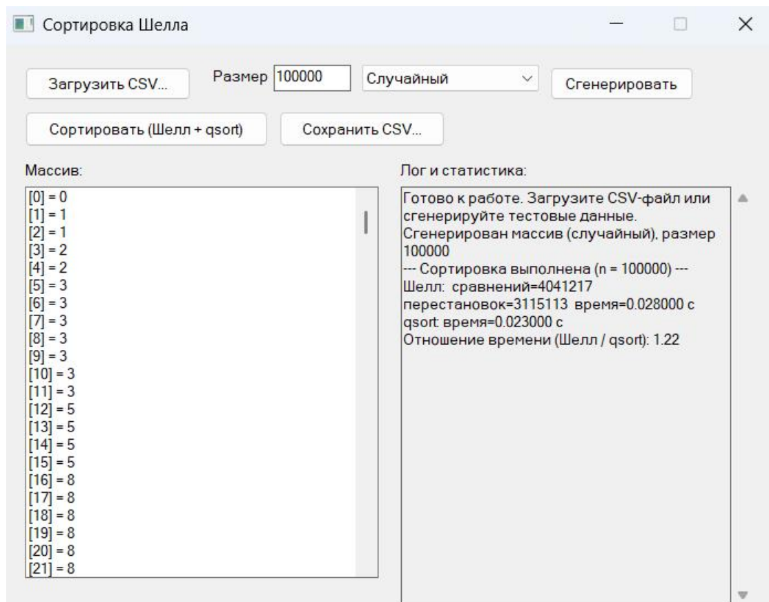
Рисунок 13 – Прогон 100000
