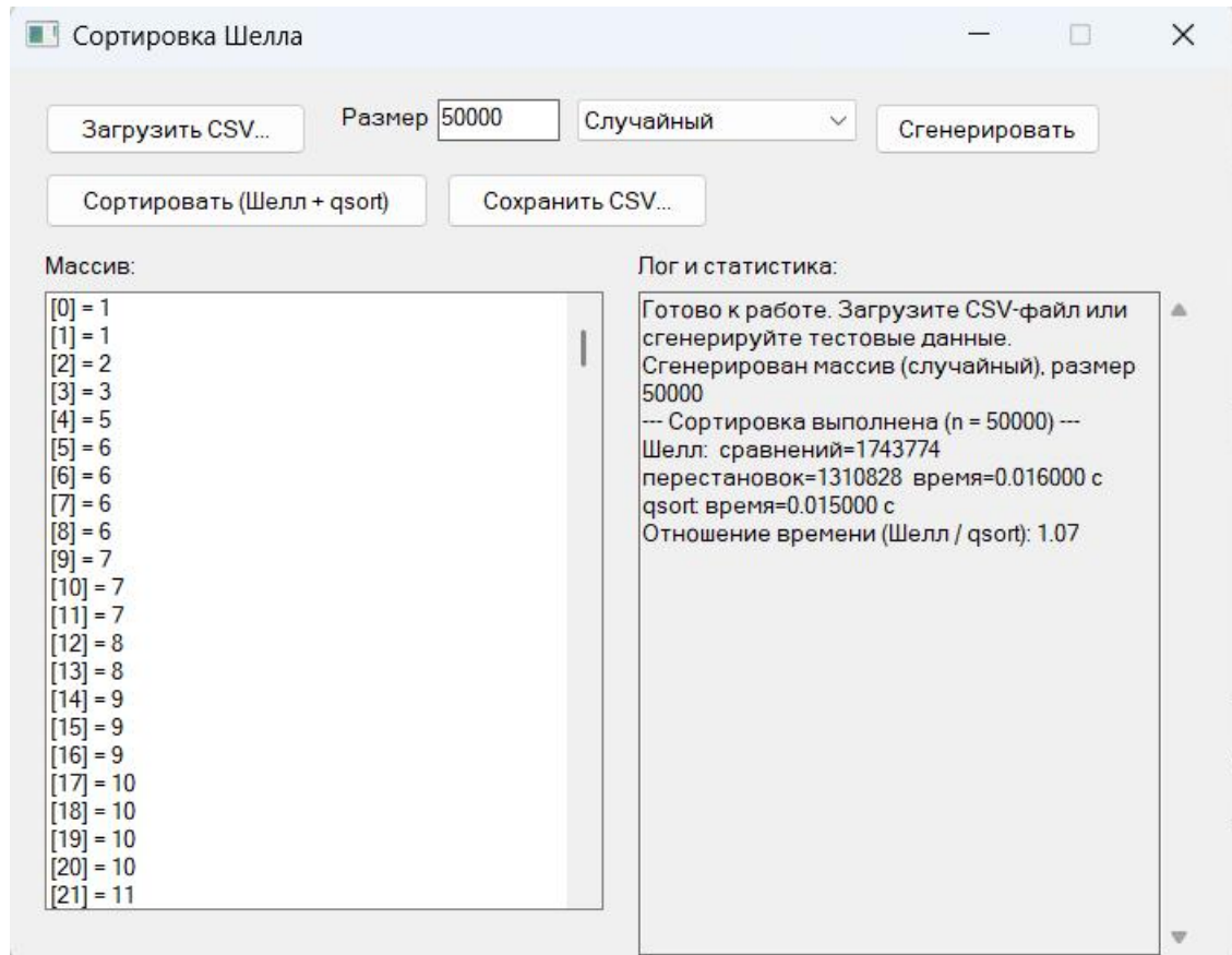
Рисунок 8 – Прогон 50000
