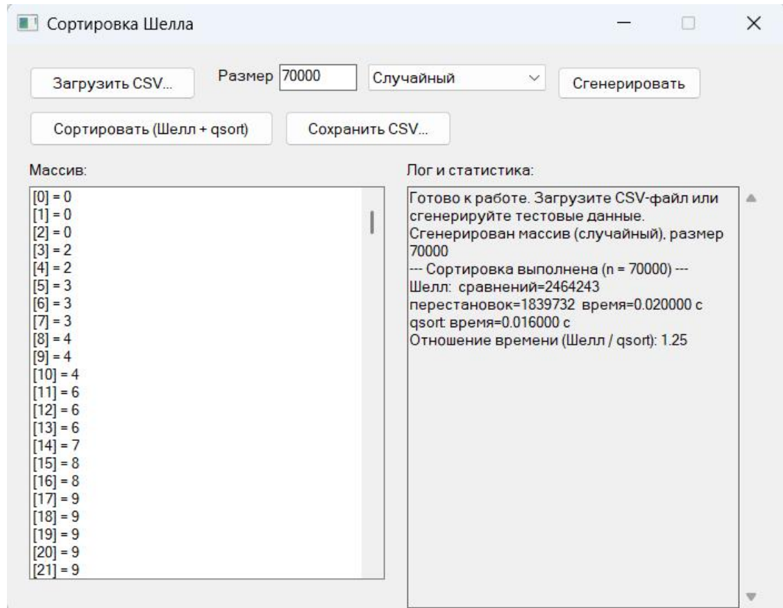
Рисунок 10 – Прогон 70000
