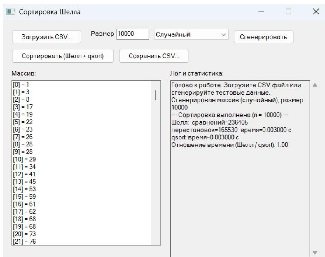
Рисунок 4 – Прогон 10000
