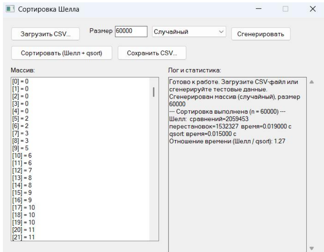
Рисунок 9 – Прогон 60000
