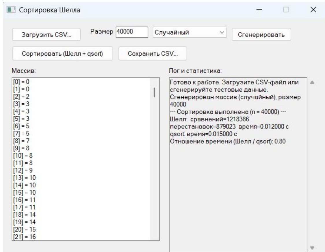
Рисунок 7 – Прогон 40000
