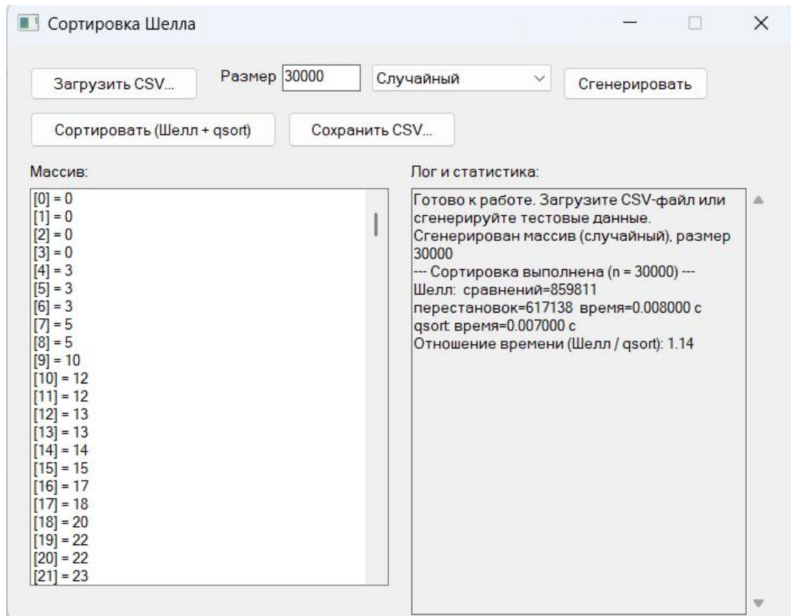
Рисунок 6 – Прогон 30000
