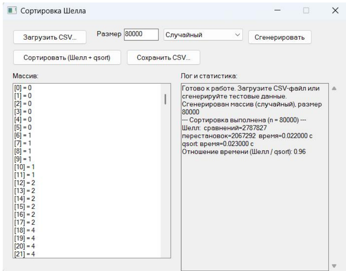
Рисунок 11 – Прогон 80000
