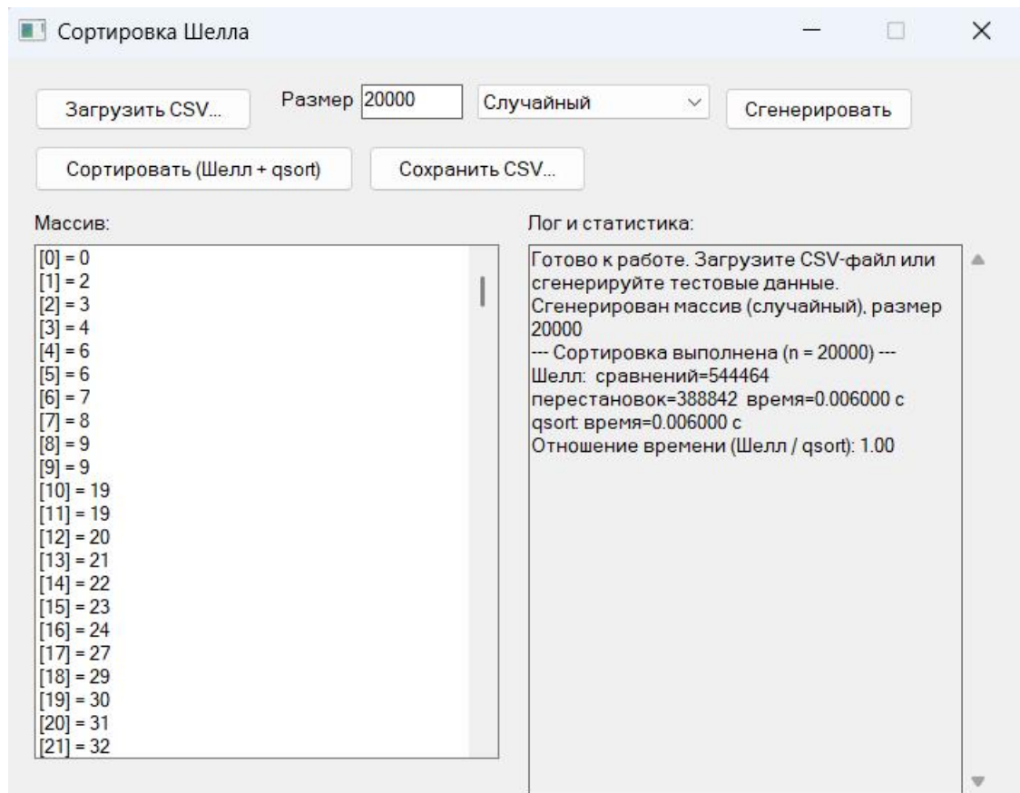
Рисунок 5 – Прогон 20000
