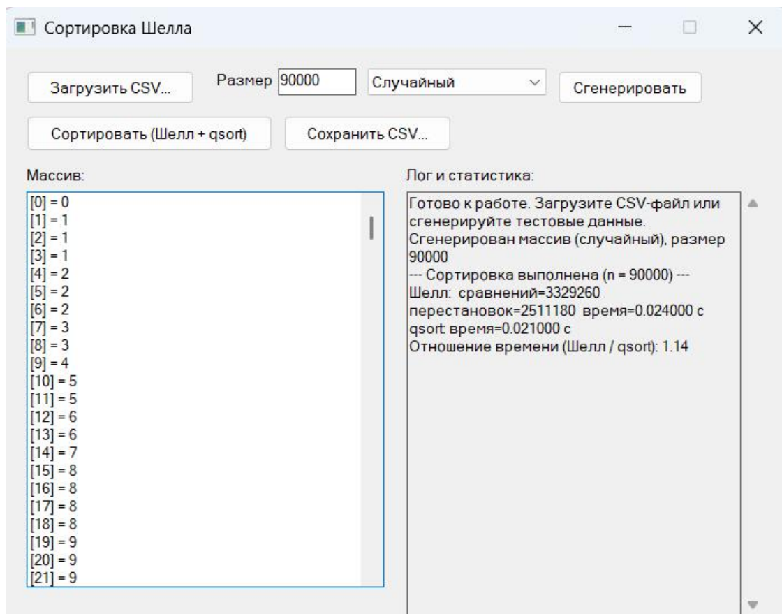
Рисунок 12 – Прогон 90000
