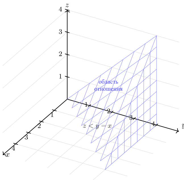
Рис. 3.2: Графическое представление отношения z < y - x, x, y, z \geq 0
