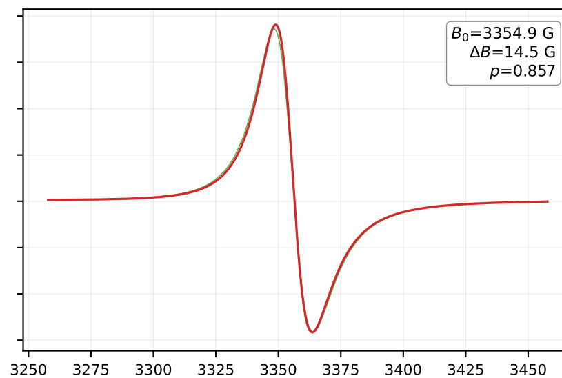
EasySpin (esfit)
